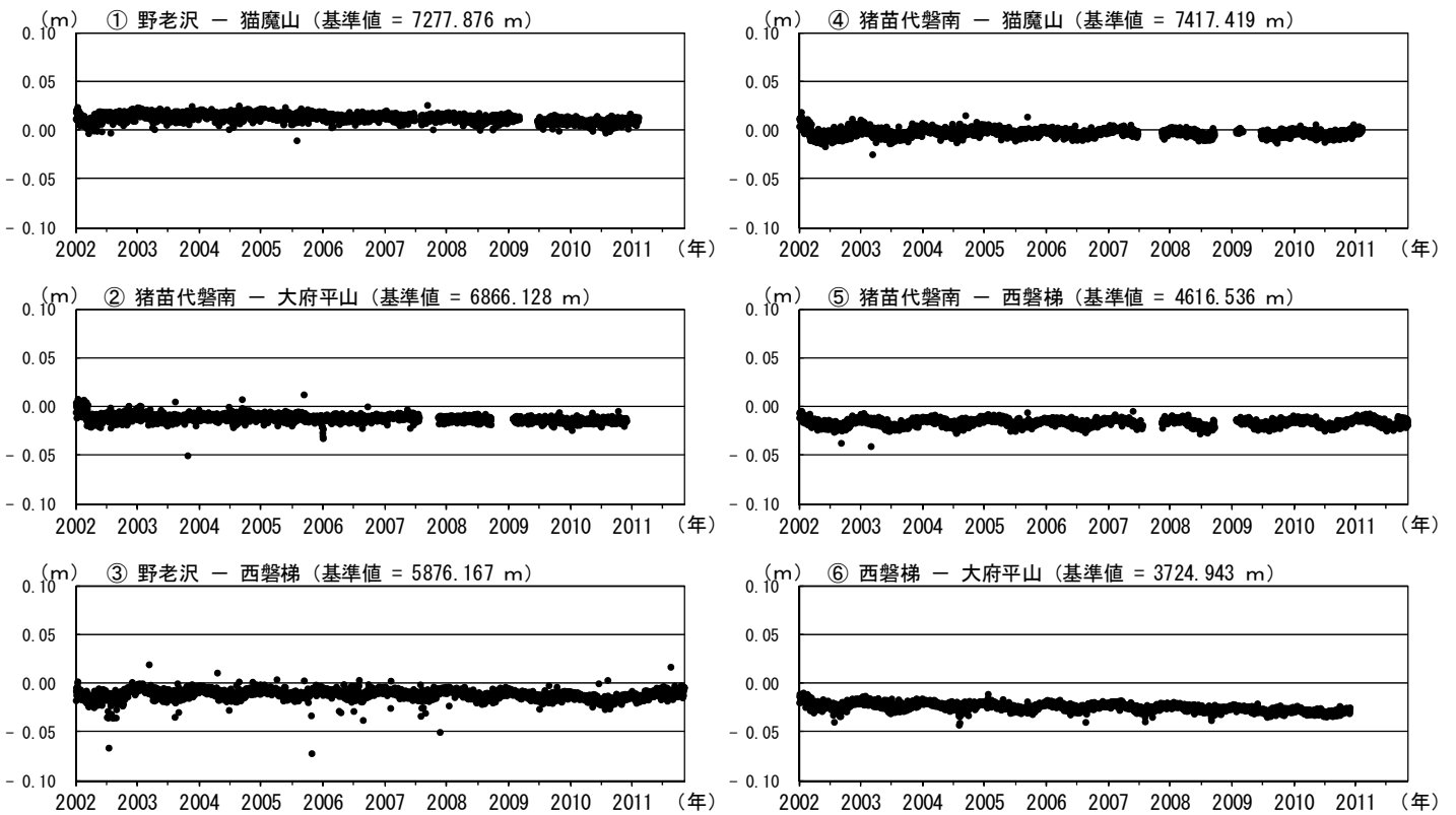
図 12 磐梯山 GPS 基線長変化図 (2002 年 1 月～2011 年 10 月)
