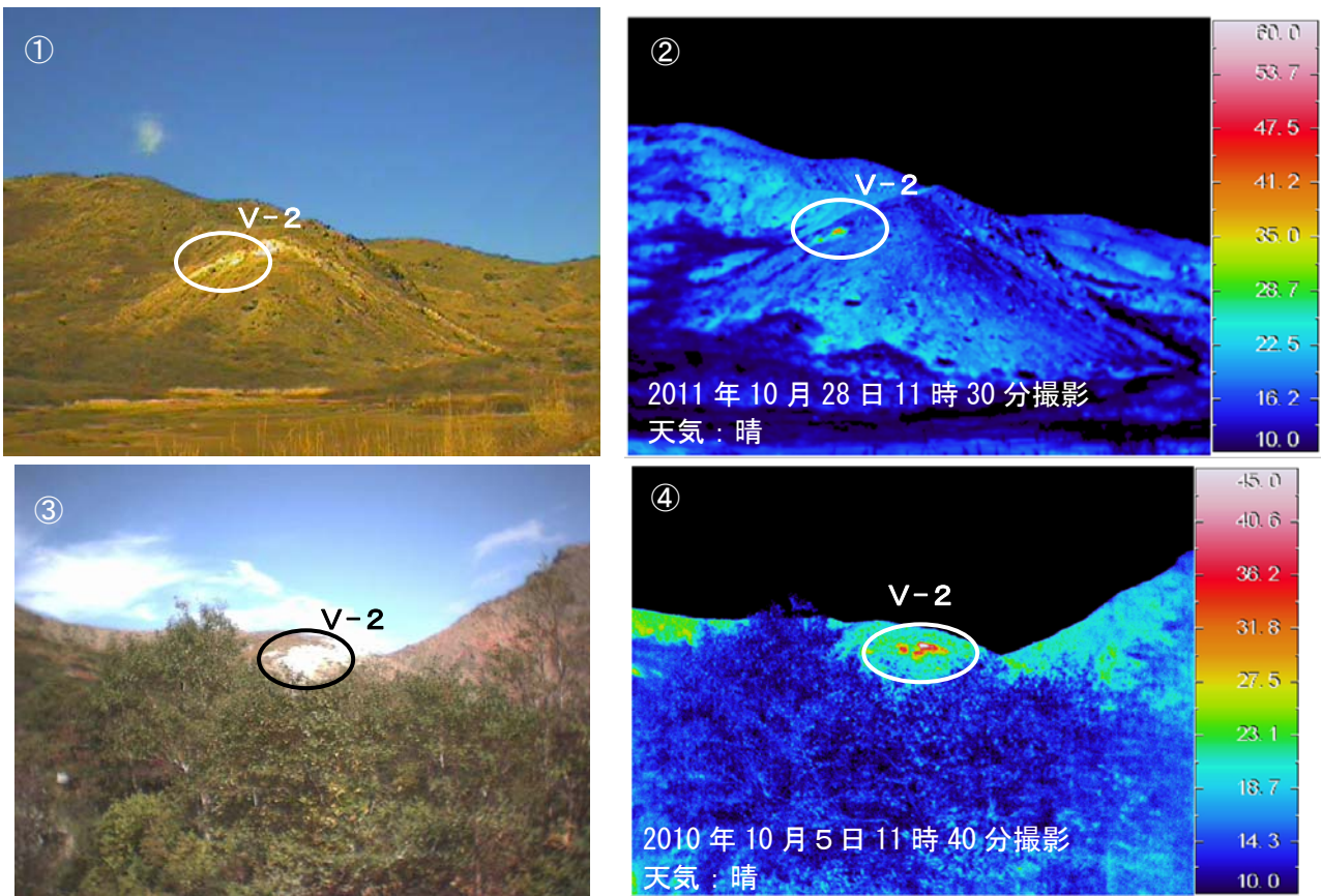
図7 磐梯山 沼ノ平(V-2)の可視画像(左)と地表面温度分布 1) (右) ①、② : 2011年10月28日撮影 ③、④ : 2010年10月5日撮影
