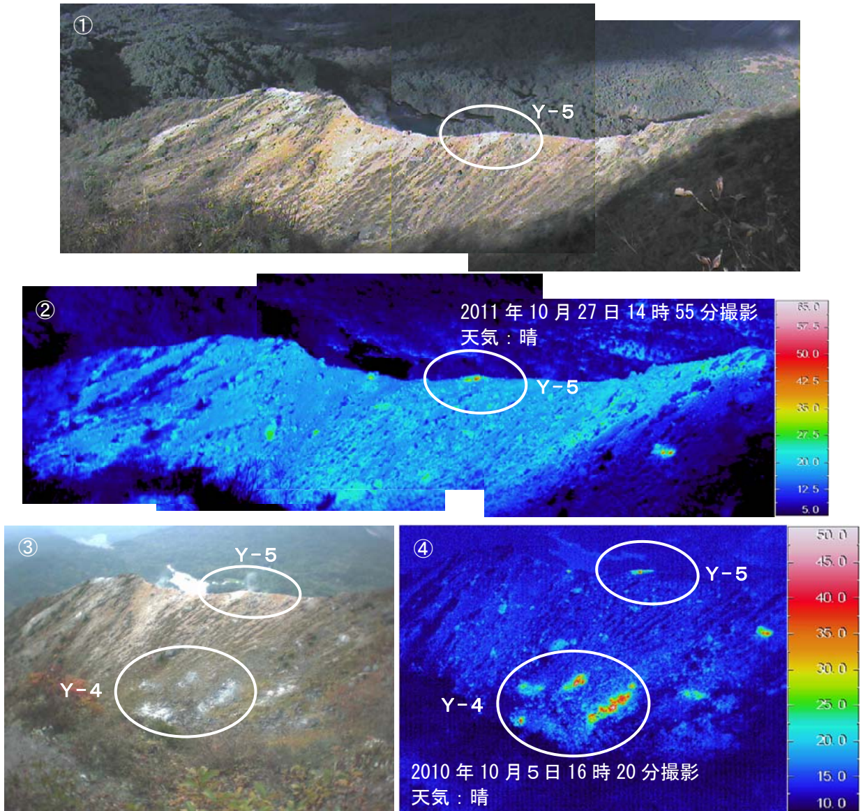
図5 磐梯山 火口壁噴気地帯 (Y-4、Y-5) の可視画像と地表面温度分布 1)
