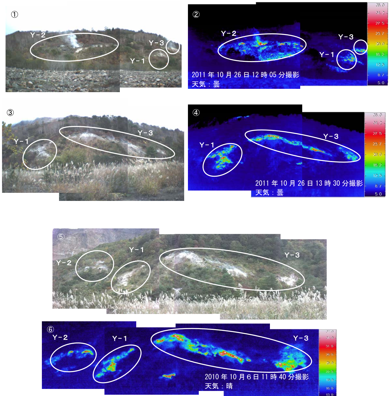
図6 磐梯山 火口壁噴気地帯 (Y-1、Y-2、Y-3) の可視画像と地表面温度分布 1) ①、②、③、④：2011年10月26日撮影 ⑤、⑥：2010年10月6日撮影
