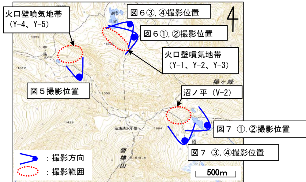
図4 磐梯山 観測ポイントと図5、6、7の撮影位置
