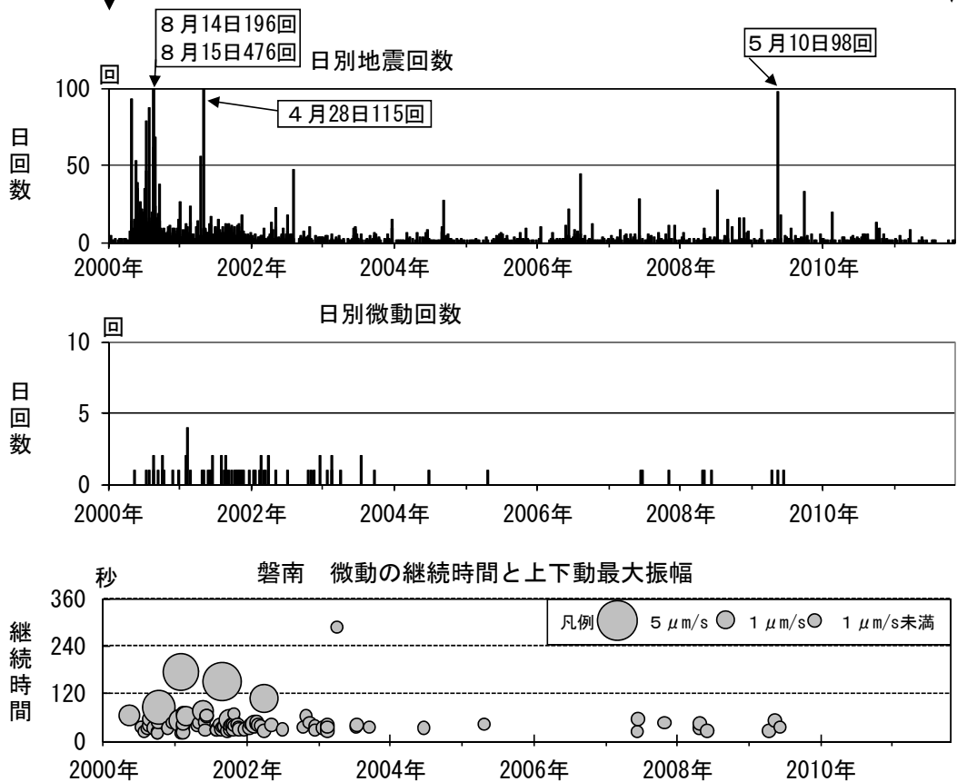
図10 磐梯山 最近の地震と微動の活動経過図 (2000年1月～2011年10月)
