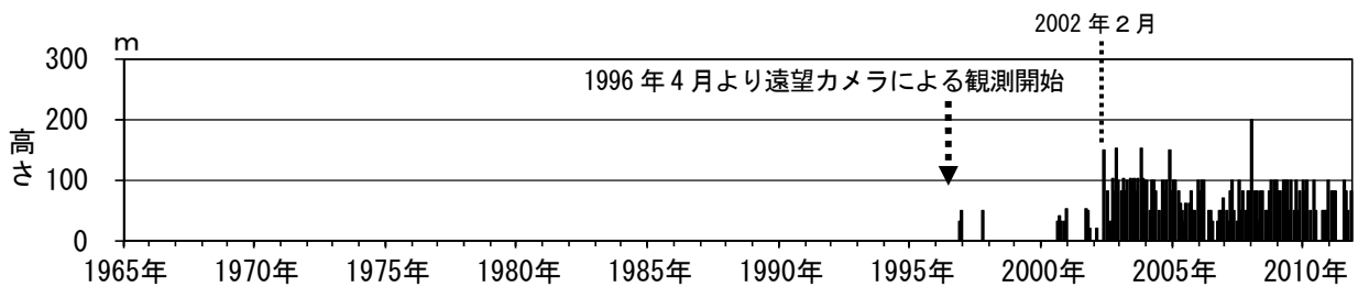
図 3 磐梯山 月最大噴気高（1996年4月～2011年10月） 2002年2月以前は定時(09時、15時)及び随時観測による高さです。 2002年2月以後は全ての時間で観測したデータによる高さです。
