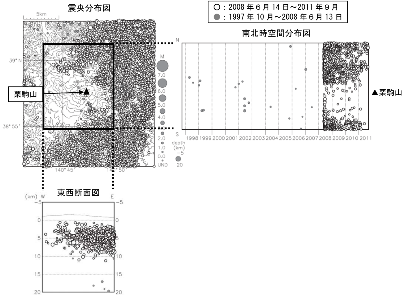
図 4 ※ 広域地震観測網による栗駒山周辺の地震活動（1997 年 10 月～2011 年 9 月）
