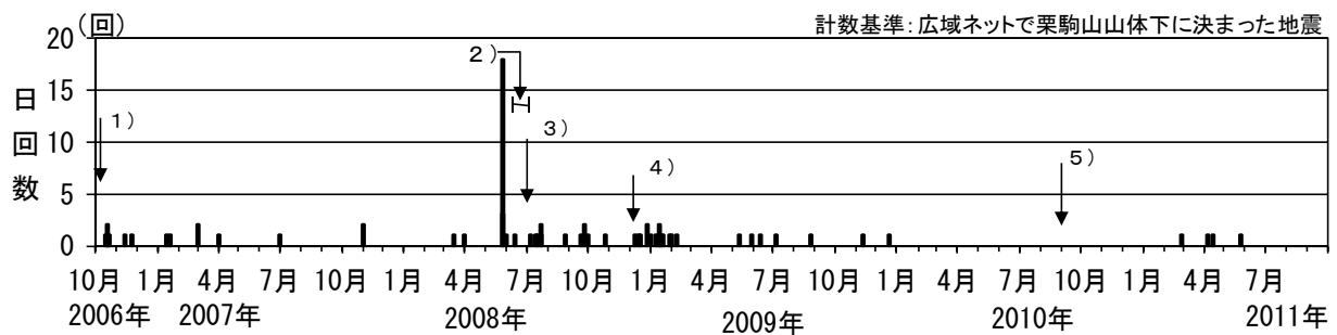
図 3※ 栗駒山 日別地震回数（2006 年 10 月～2011 年 9 月）
