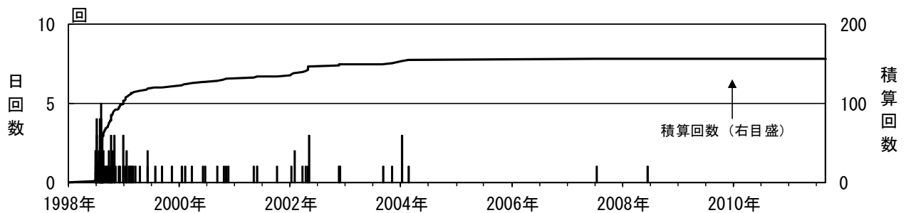
図 6※ 岩手山 日別微動回数（1998 年 1 月～2011 年 8 月）
