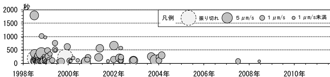
図 7※ 岩手山 微動の継続時間と上下動最大振幅（1998 年 1 月～2011 年 8 月）
