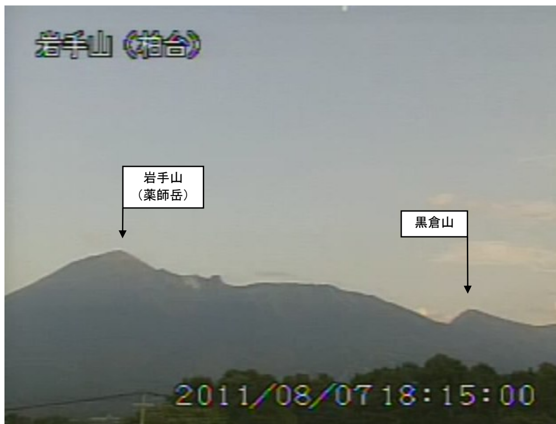
図 2 岩手山 遠望カメラの映像（8 月 7 日 18 時 15 分頃） 柏台（黒倉山山頂の北約 8 km）に設置してある遠望カメラによる。
