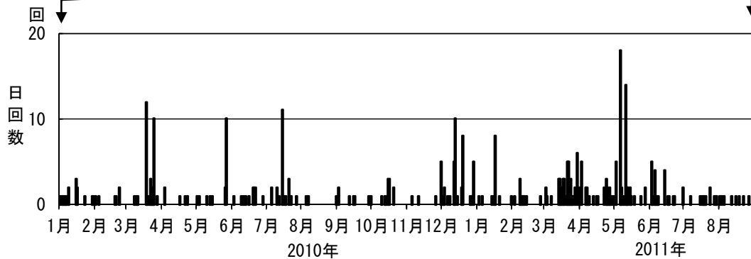
図 5※ 岩手山 日別地震回数（2010 年 1 月～2011 年 8 月）
