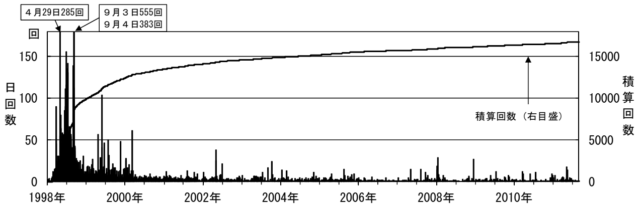
図 4※ 岩手山 日別地震回数（1998 年 1 月～2011 年 8 月）
