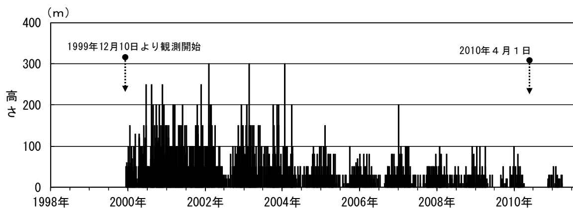
図 3 岩手山 日最大噴気の高さ（1999 年 12 月～2011 年 8 月）
