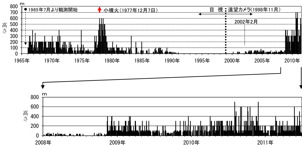
図4 吾妻山の噴気の高さ 上段：月別最大噴気（噴煙）高（1965 年 7 月～2011 年 6 月） 下段：日別最大噴気高（2008 年 1 月～2011 年 6 月）
