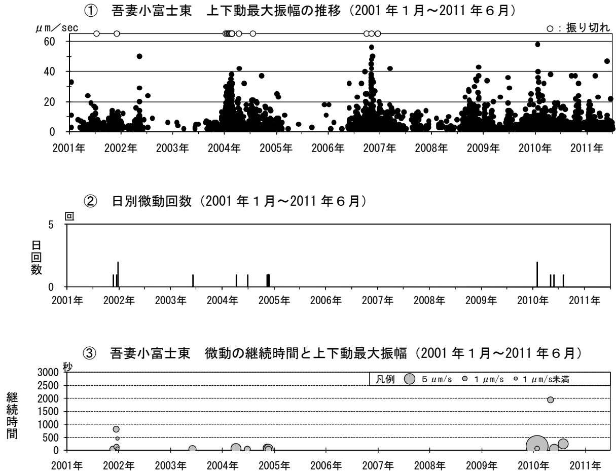
図 8 吾妻山 地震活動経過図（2）
