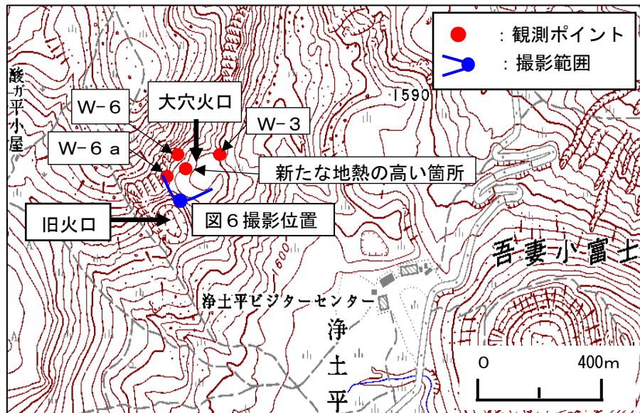
図5 吾妻山 観測ポイント及び可視画像と地表面温度分布 1) 撮影位置
