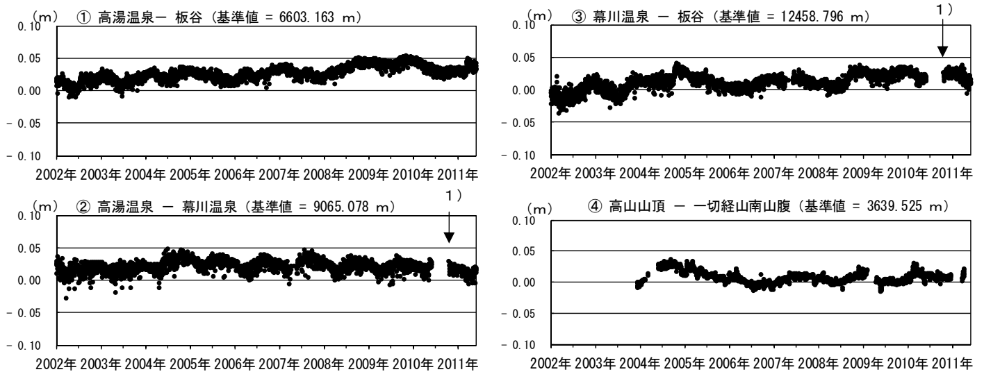
図 10 吾妻山 GPS 基線長変化図（2002 年 1 月～2011 年 6 月）
