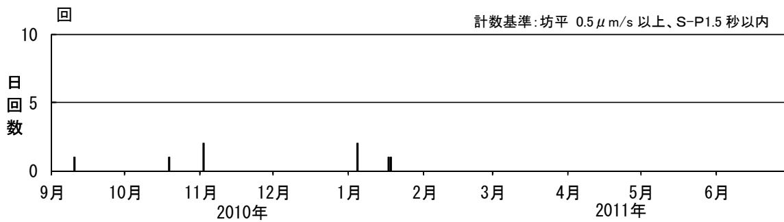
図3 蔵王山 火山性地震の日別回数（2010年9月～2011年6月）
