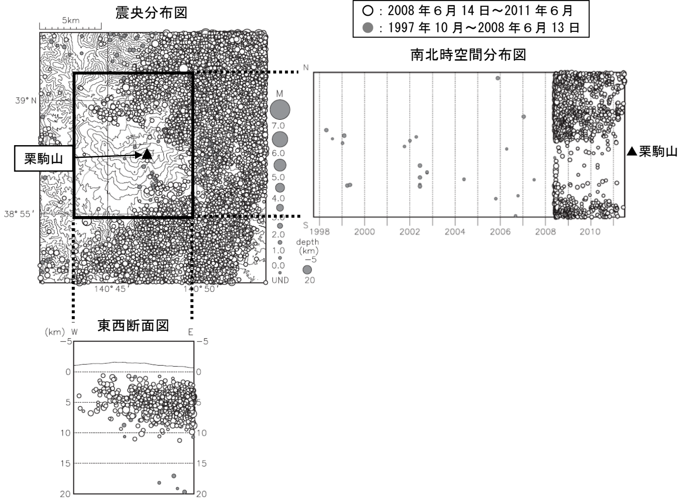
図 4※ 栗駒山周辺の地震活動（1997 年 10 月～2011 年 6 月）
