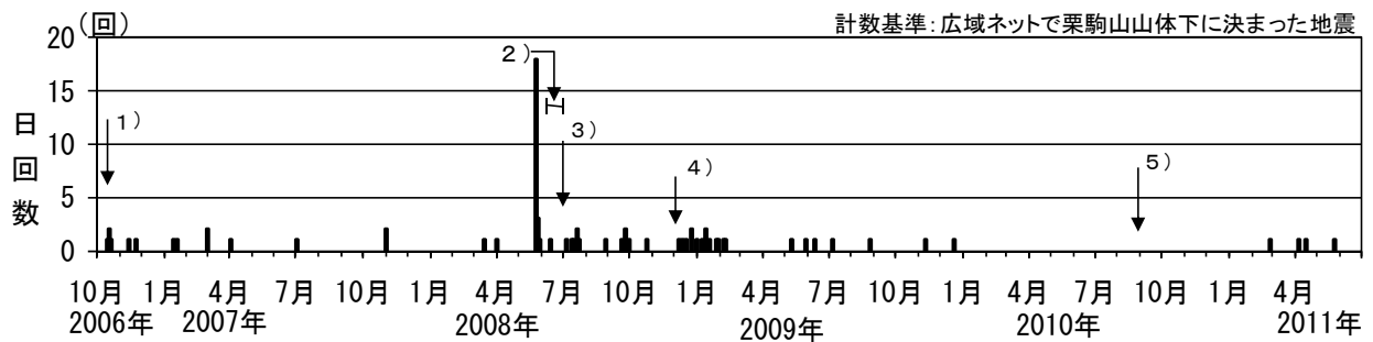
図3※ 栗駒山 日別地震回数（2006年10月～2011年6月）
