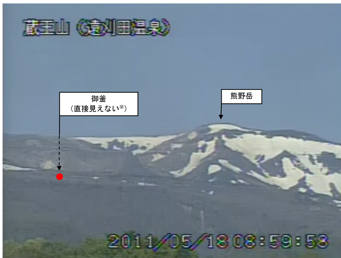
図 2 蔵王山 遠望カメラの映像（5 月 18 日 09 時 00 分頃）
