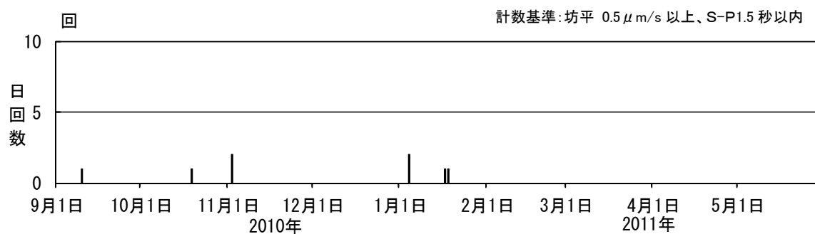
図 3 蔵王山 火山性地震の日別回数（2010 年 9 月～2011 年 5 月）
