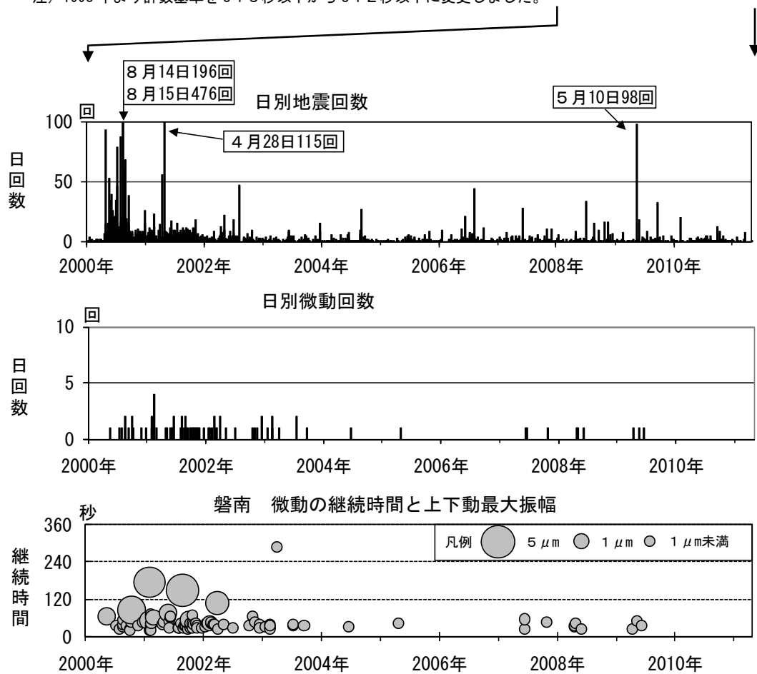
図 5 磐梯山 最近の地震と微動の活動経過図（2000 年 1 月～2011 年 4 月）
