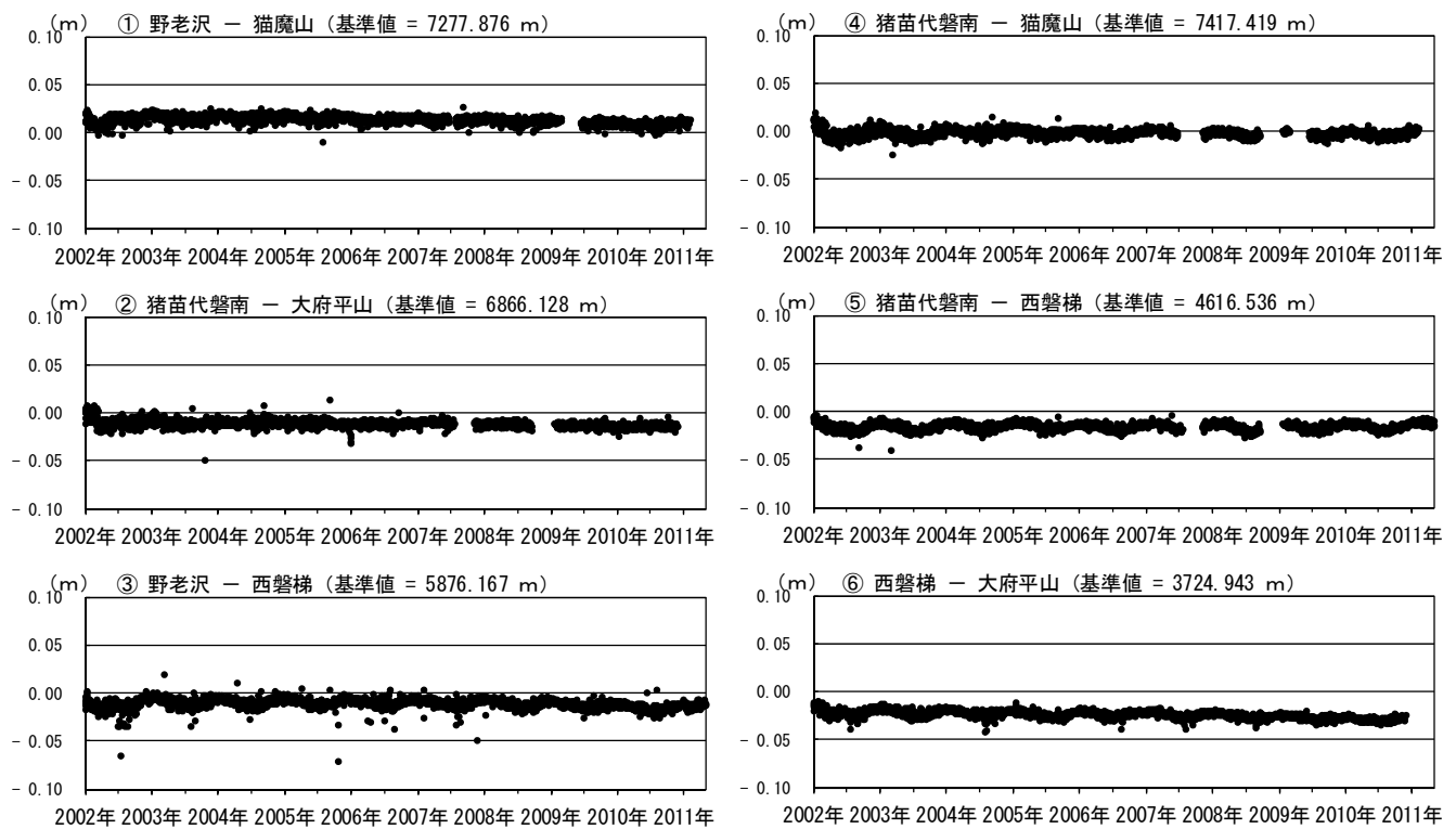
図 7 磐梯山 GPS 基線長変化図（2002 年 1 月～2011 年 4 月）
