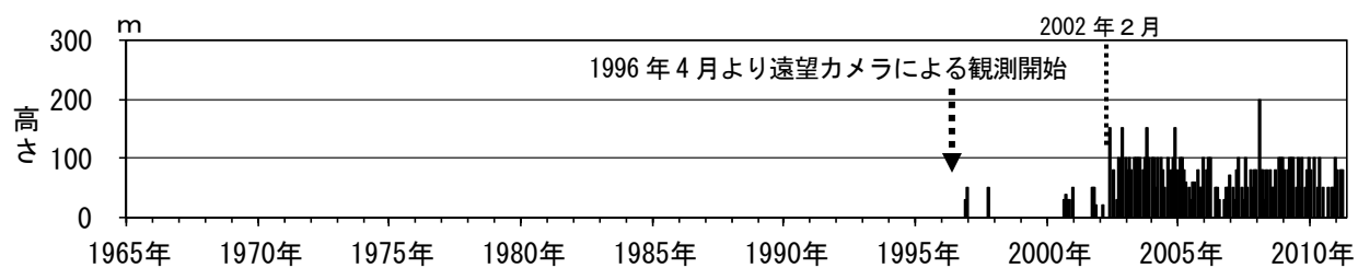
図3 磐梯山 月最大噴気高（1996年4月～2011年4月） 2002年2月以前は定時(09時、15時)及び随時観測による高さです。 2002年2月以後は全ての時間で観測したデータによる高さです。
