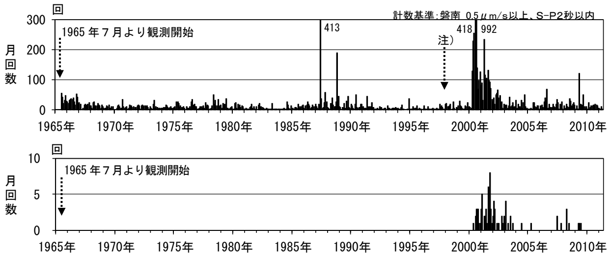
図 4 磐梯山 上段：月別地震回数(1965 年 7 月～2011 年 4 月)
