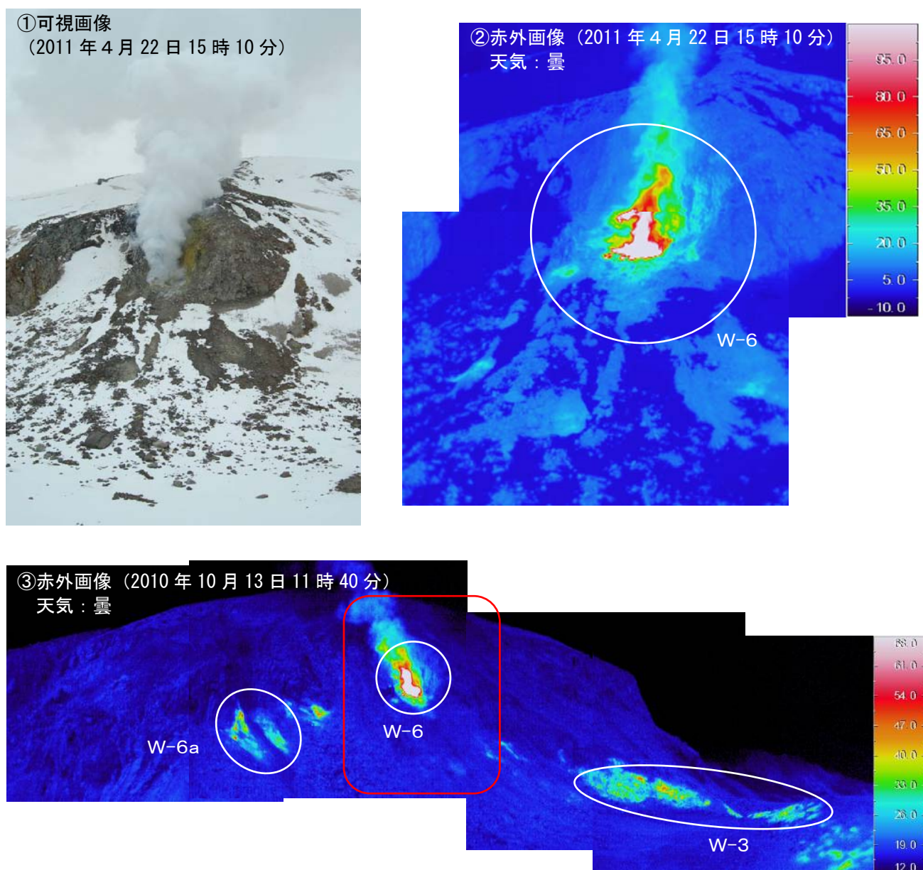
図 8 吾妻山 大穴火口内北壁の可視画像と地表面温度分布 1)
