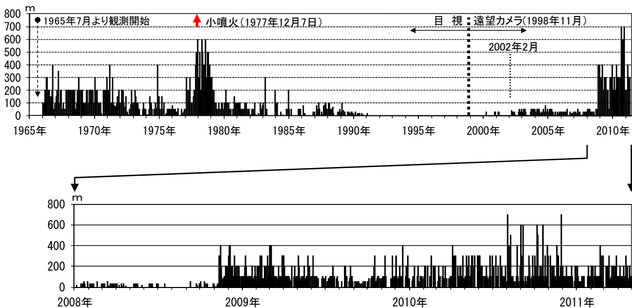
図4 吾妻山の噴気の高さ 上段：月別最大噴気（噴煙）高（1965 年 7 月～2011 年 4 月） 下段：日別最大噴気高（2008 年 1 月～2011 年 4 月）
