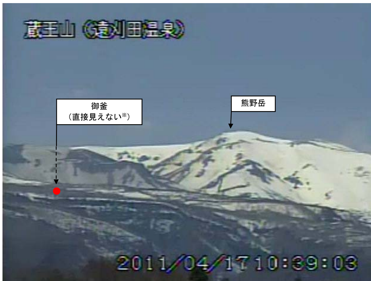
図2 蔵王山 遠望カメラの映像（4月17日10時39分頃）
