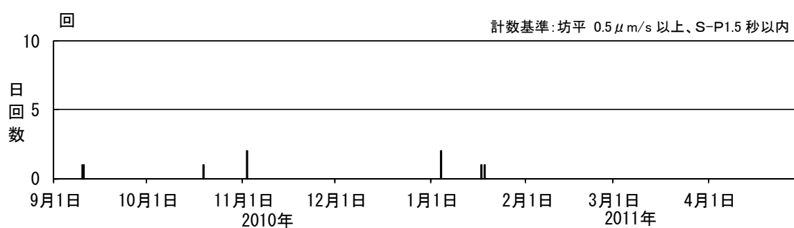
図3 蔵王山 火山性地震の日別回数（2010年9月～2011年4月）
