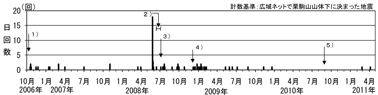
図3※ 栗駒山 日別地震回数（2006年10月～2011年4月）
