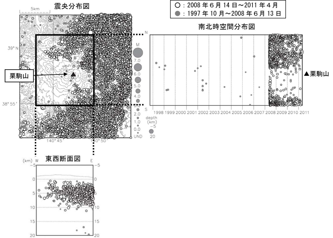
図 4※ 栗駒山周辺の地震活動（1997 年 10 月～2011 年 4 月）
