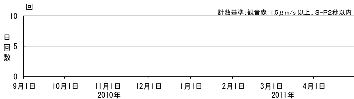
図3 鳥海山 火山性地震の日別回数（2010年9月～2011年4月）
