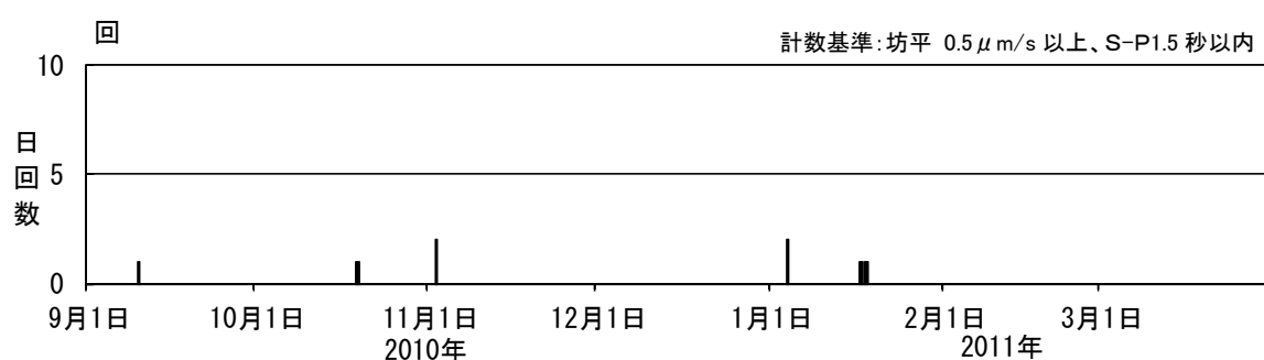
図3 蔵王山 火山性地震の日別回数（2010年9月～2011年3月）
