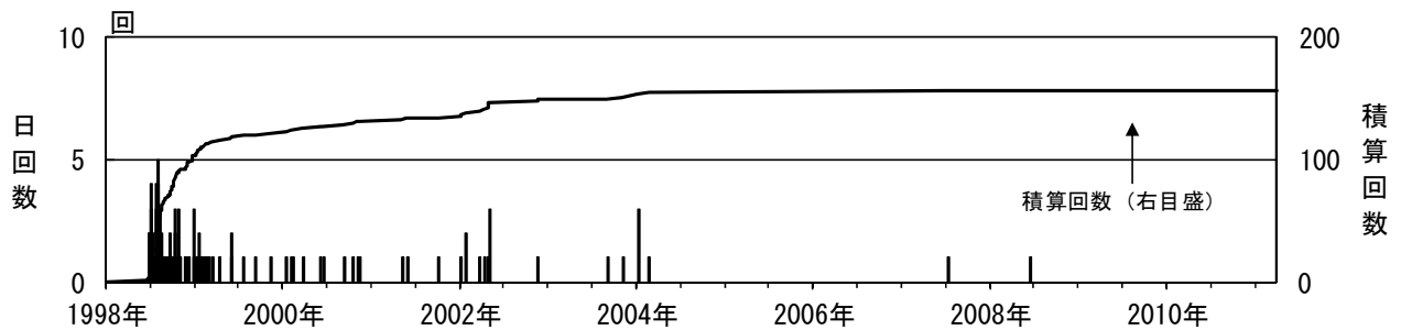
図 6※ 岩手山 日別微動回数（1998 年 1 月～2011 年 3 月）
