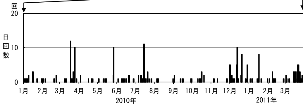
図 5※ 岩手山 日別地震回数（2010 年 1 月～2011 年 3 月）
