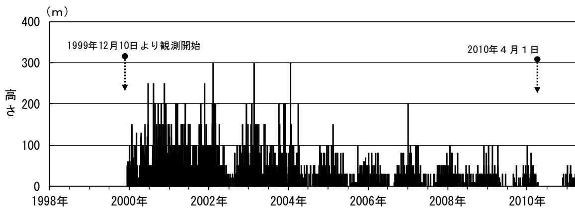
図 3 岩手山 日最大噴気の高さ（1999年12月～2011年3月） 柏台遠望カメラで、1999年12月10日より観測を開始しています。 2010年3月までは、黒倉山のみを観測していましたが、2010年4月1日より、岩手山全体を観測しています。
