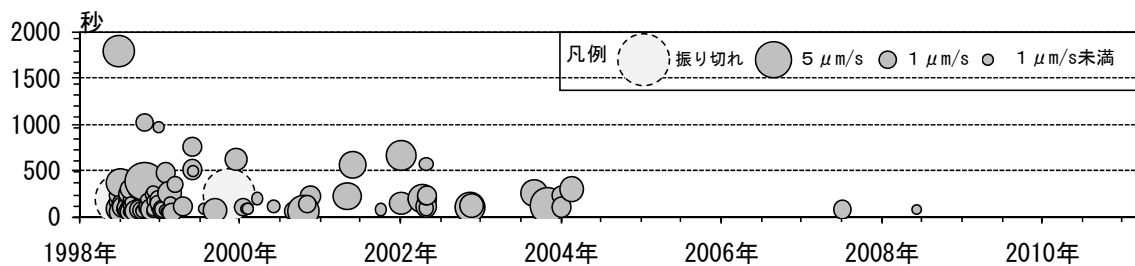
図 7※ 岩手山 微動の継続時間と上下動最大振幅（1998 年 1 月～2011 年 3 月）
