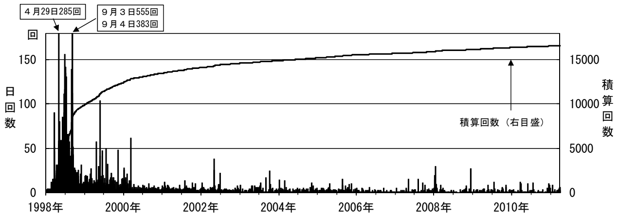
図 4※ 岩手山 日別地震回数（1998 年 1 月～2011 年 3 月）
