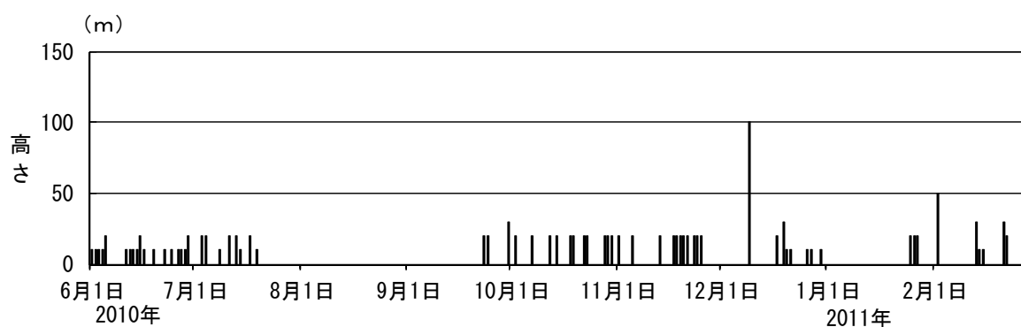
図 3※ 秋田焼山 日別最大噴気の高さ（2010 年 6 月～2011 年 2 月）
