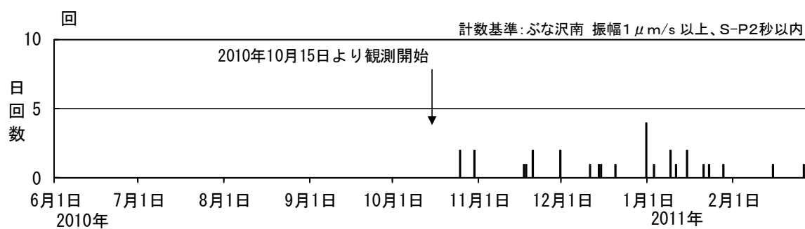
図 4 秋田焼山 火山性地震の日別回数（2010 年 10 月～2011 年 2 月）
