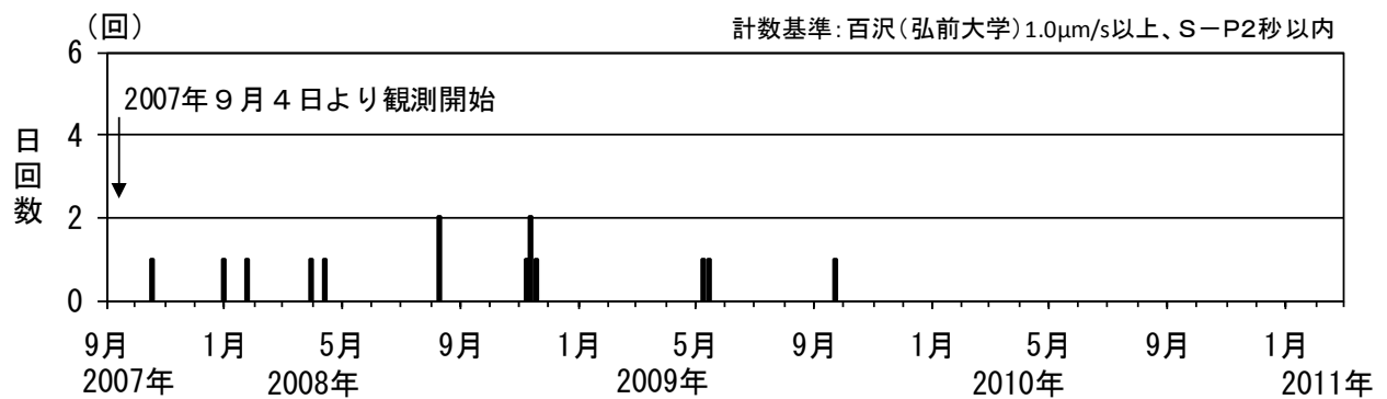
図3※ 岩木山 日別地震回数（2007年9月～2011年2月） 弘前大学からのデータ提供により、2007年9月4日から観測を開始しています。
