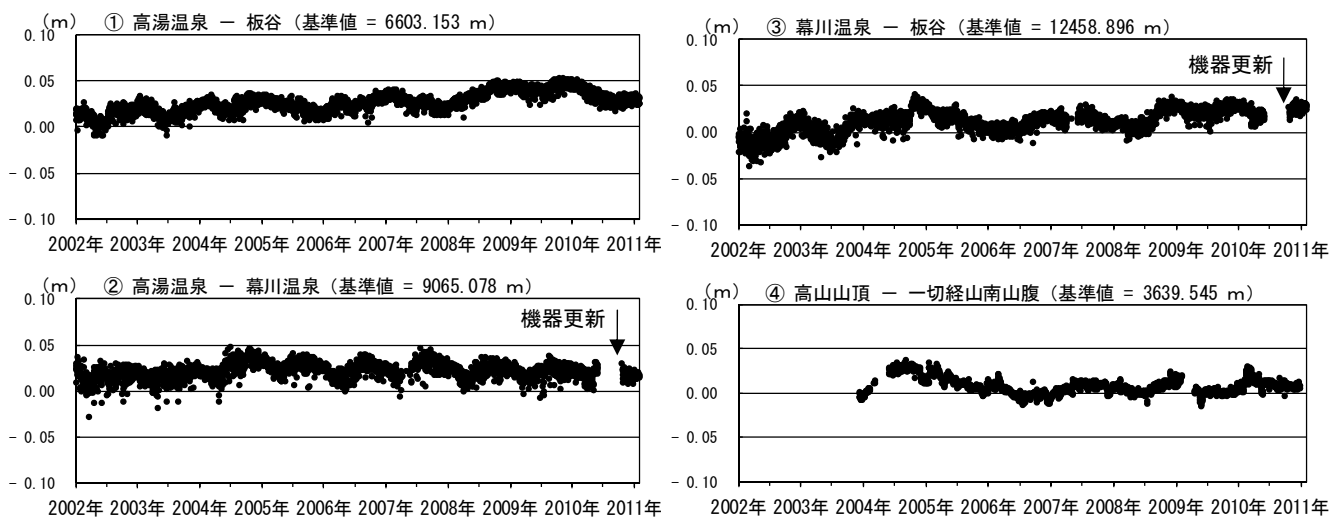
図 6 吾妻山 GPS 基線長変化図（2002 年 1 月～2011 年 1 月）
