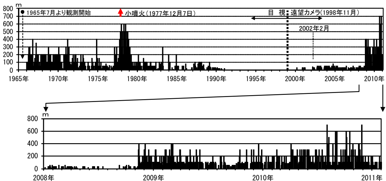
図3 吾妻山の噴気の高さ 上段：月別最大噴気（噴煙）高（1965年7月～2011年1月） 下段：日別最大噴気高（2008年1月～2011年1月） 1998年以前は福島地方气象台（大穴火口の東北東約20km）からの目視観測です。 1998年から遠望カメラ（大穴火口の東北東約14km）による観測です。 2002年2月以前は定時（09時、15時）及び随時観測による高さです。 2002年2月以後は全ての時間で観測したデータによる高さです。 2010年8月3日、11月27日に一時的に700m、8月31日、9月5日、10月6日、10月18日に一時的に600mを観測しました。
