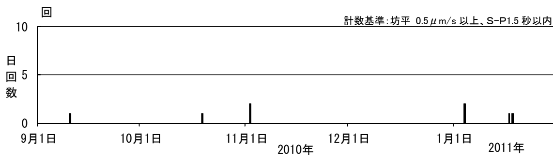
図 3 蔵王山 火山性地震の日別回数（2010 年 9 月～2011 年 1 月）
