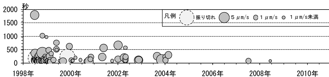
図 6※ 岩手山 微動の継続時間と上下動最大振幅（1998 年 1 月～2011 年 1 月）
