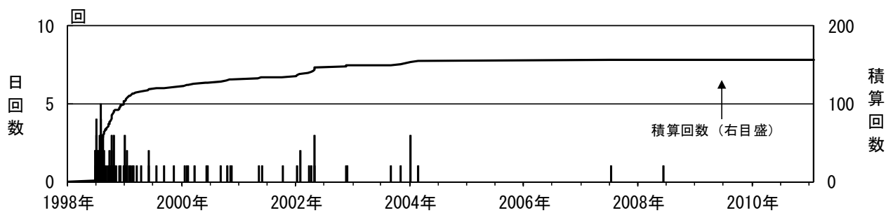
図 5※ 岩手山 日別微動回数（1998 年 1 月～2011 年 1 月）
