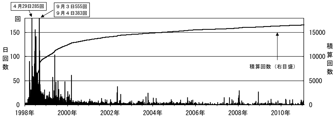
図 4※ 岩手山 日別地震回数（1998 年 1 月～2011 年 1 月）
