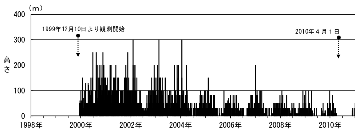
図 3 岩手山 日最大噴気の高さ（1999 年 12 月～2011 年 1 月） 柏台遠望カメラで、1999 年 12 月 10 日より観測を開始しています。 2010 年 3 月までは、黒倉山のみを観測していましたが、2010 年 4 月 1 日より、岩手山全体を観測しています。
