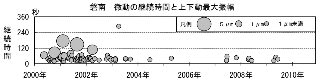
図4 磐梯山 最近の地震と微動の活動経過図（2000年1月～2010年11月）
