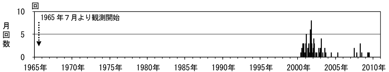
図3 磐梯山 上段：月別地震回数（1965年7月～2010年11月）
