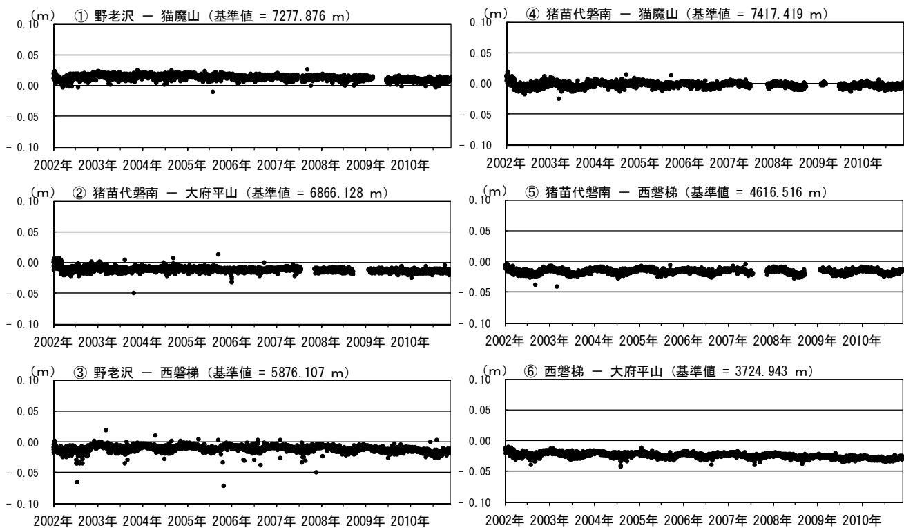
図 6 磐梯山 GPS 基線長変化図（2002 年 1 月～2010 年 11 月）
