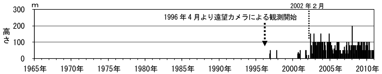
図2 磐梯山 月最大噴気高（1996年4月～2010年11月）
