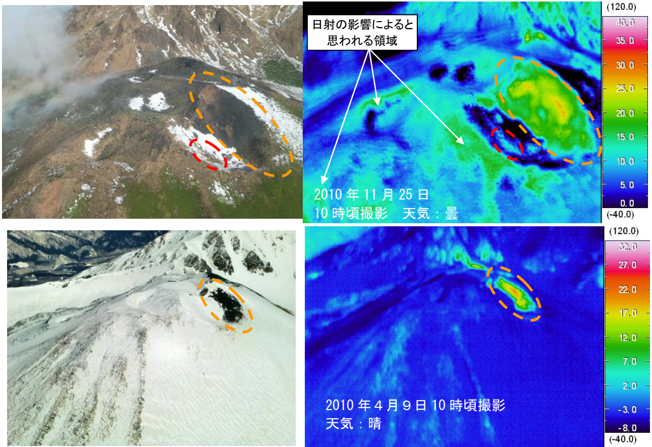
図7 秋田駒ヶ岳 女岳南東火口付近の可視画像（上）と地表面温度分布 1) （下） 上段：2010年11月25日撮影（岩手県の協力により上空から撮影） 下段：2010年4月9日撮影（岩手県の協力により上空から撮影） ・図の破線橙色丸囲みの領域が、2010年6月に確認された地熱の高い箇所です。 4月9日の地表面温度分布 1) でも高く表現されています。 ・図の破線赤丸囲みの領域が、2010年10月に確認された地熱の高い箇所です。
