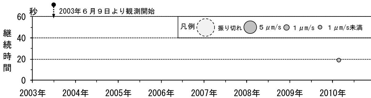
図3※ 秋田駒ヶ岳 微動の継続時間と上下動最大振幅（2003年6月～2010年11月） 東北大学秋田駒ヶ岳観測点による。
