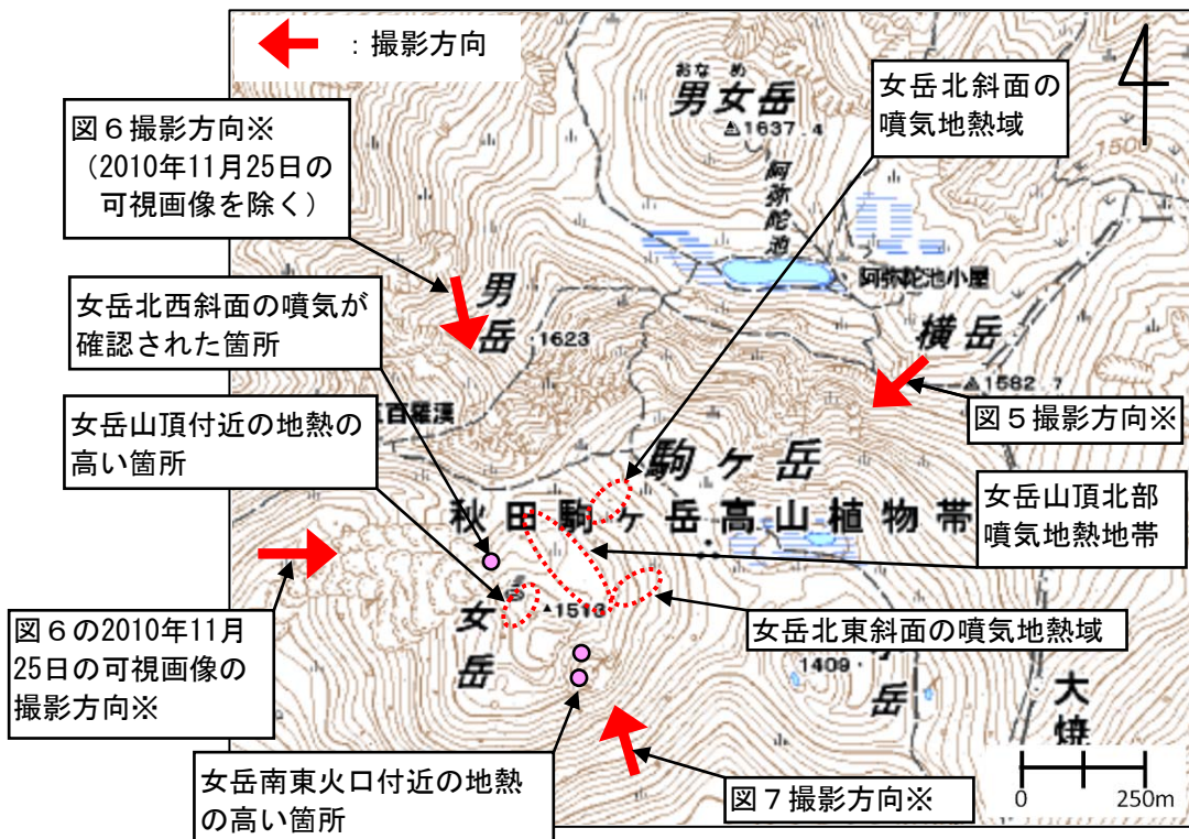
図4 秋田駒ヶ岳 地形図と図5～7の撮影方向
