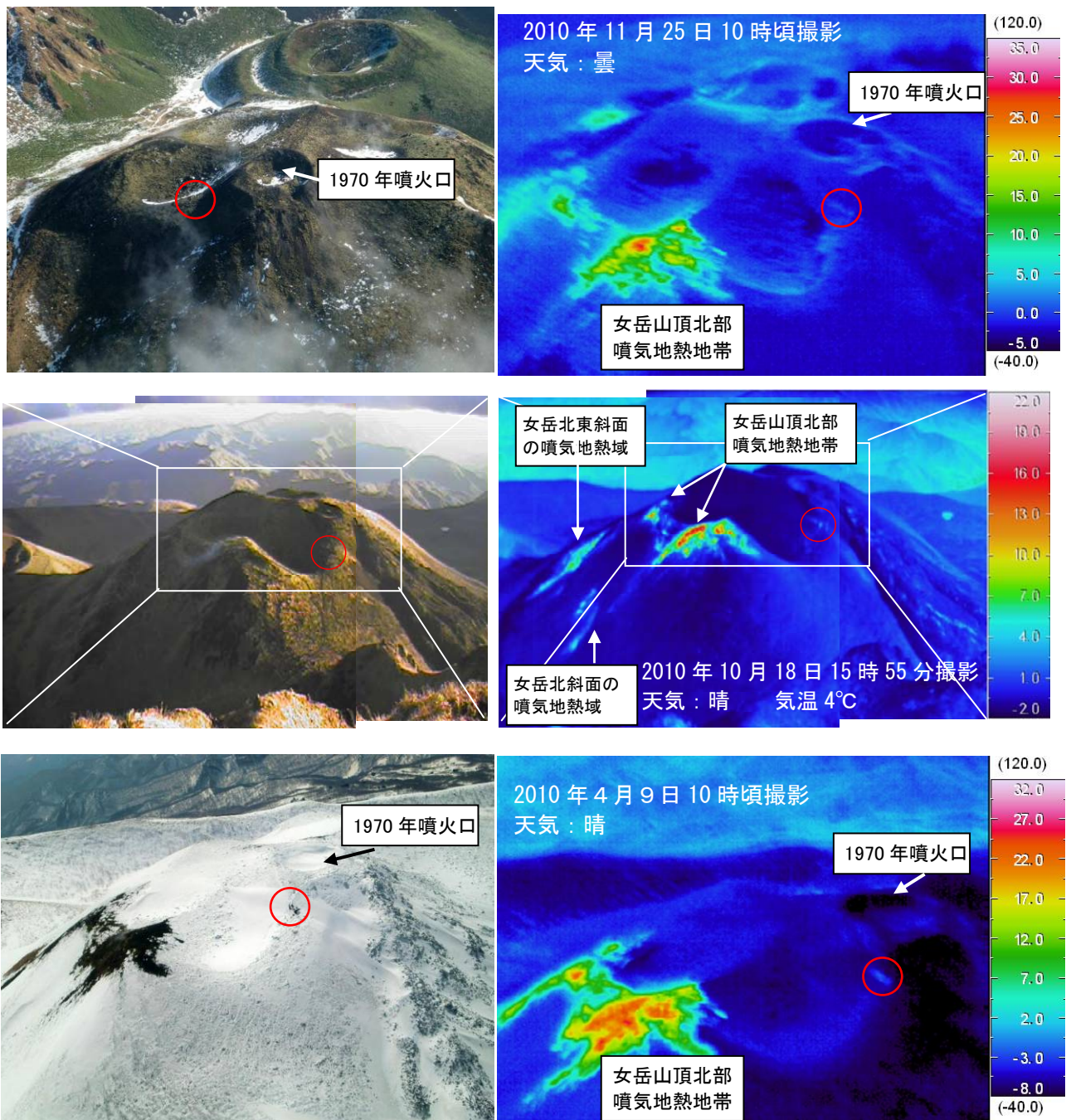
図6 秋田駒ヶ岳 女岳の可視画像（左）と地表面温度分布 1) （右） 1 段目：2010年11月25日撮影（岩手県の協力により上空から撮影） 2 段目：2010年10月18日撮影 3 段目：2010年4月9日撮影（岩手県の協力により上空から撮影） ・図の赤丸が、2010年10月18日の現地調査で噴気を確認した箇所です。
