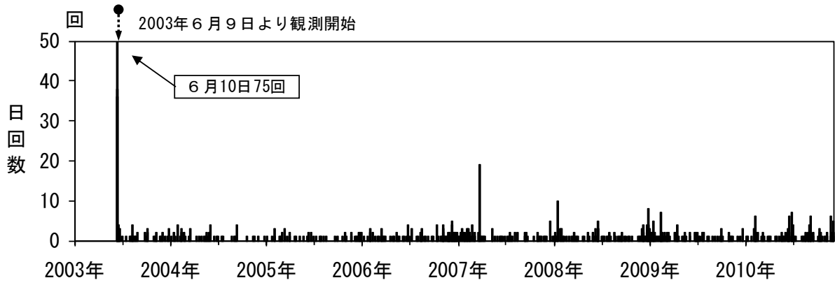
図2※ 秋田駒ヶ岳 日別地震回数（2003年6月～2010年11月）
