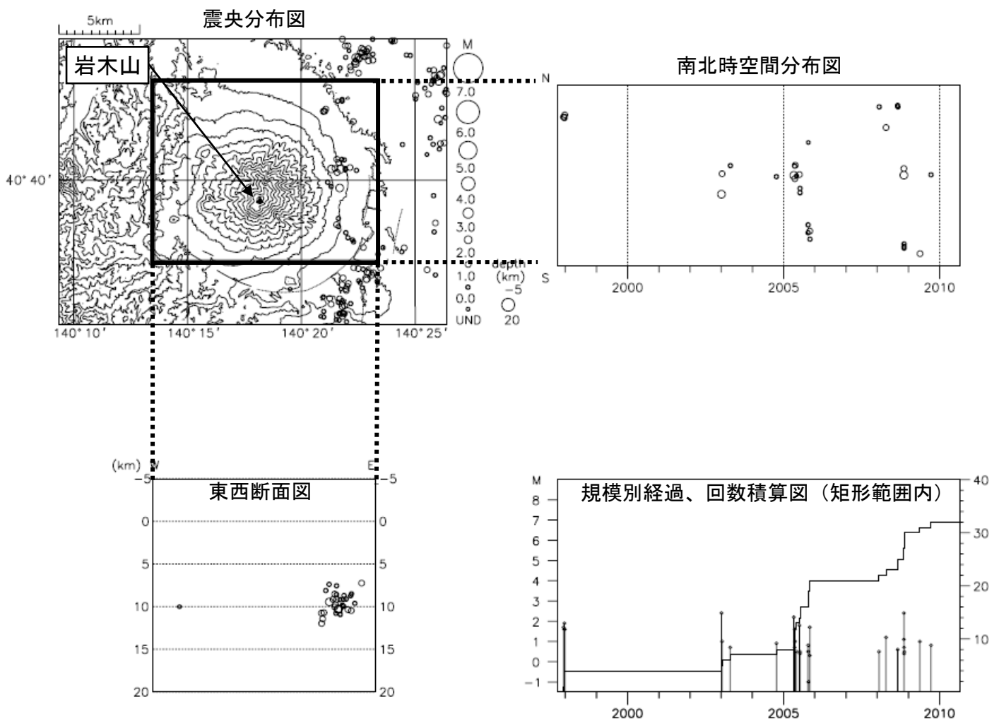
図 3※ 岩木山周辺の地震活動（1997 年 10 月～2010 年 8 月）
