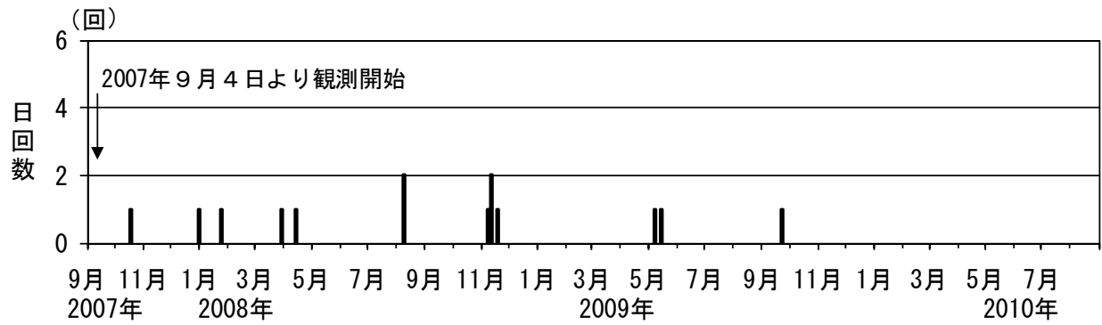
図 2※ 岩木山 日別地震回数（2007 年 9 月～2010 年 8 月）
