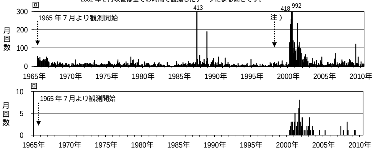
図3 磐梯山 上段：月別地震回数(1965 年 7 月～2010 年 6 月)
