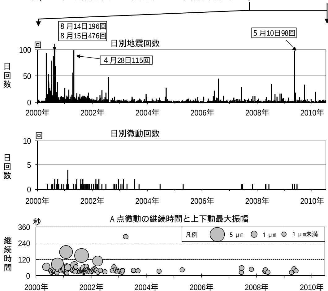
図4 磐梯山 最近の地震と微動の活動経過図（2000 年 1 月～2010 年 6 月）
