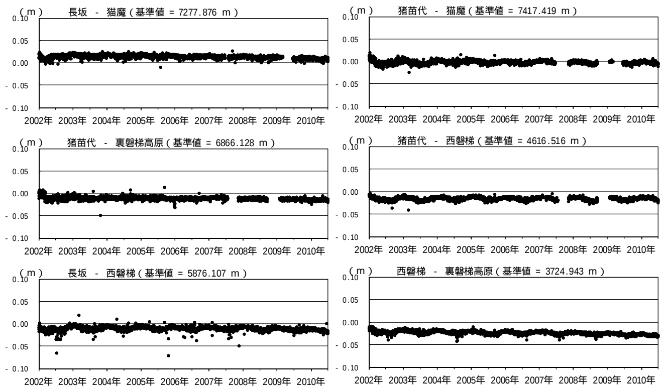
図6 磐梯山 GPS 基線長変化図（2002 年 1 月～2010 年 6 月）
