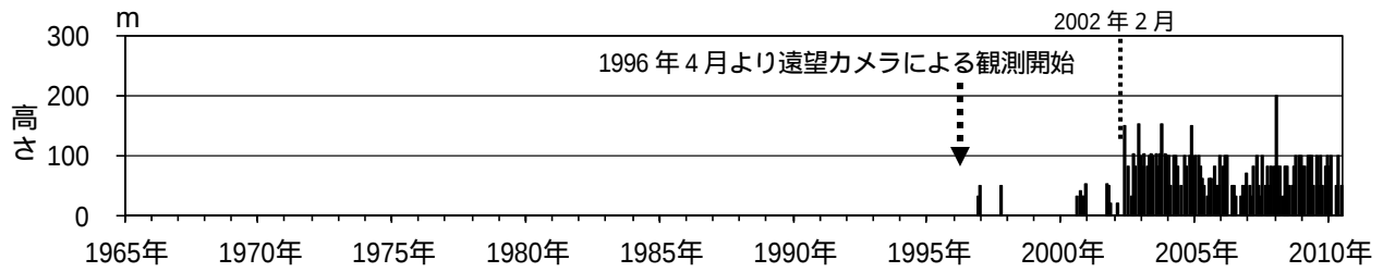
図2 磐梯山 月最大噴気高（1996 年 4 月～2010 年 6 月）
