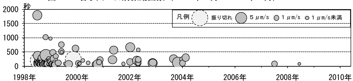
図 6※ 岩手山 微動の継続時間と上下動最大振幅（1998 年 1 月～2010 年 5 月）
