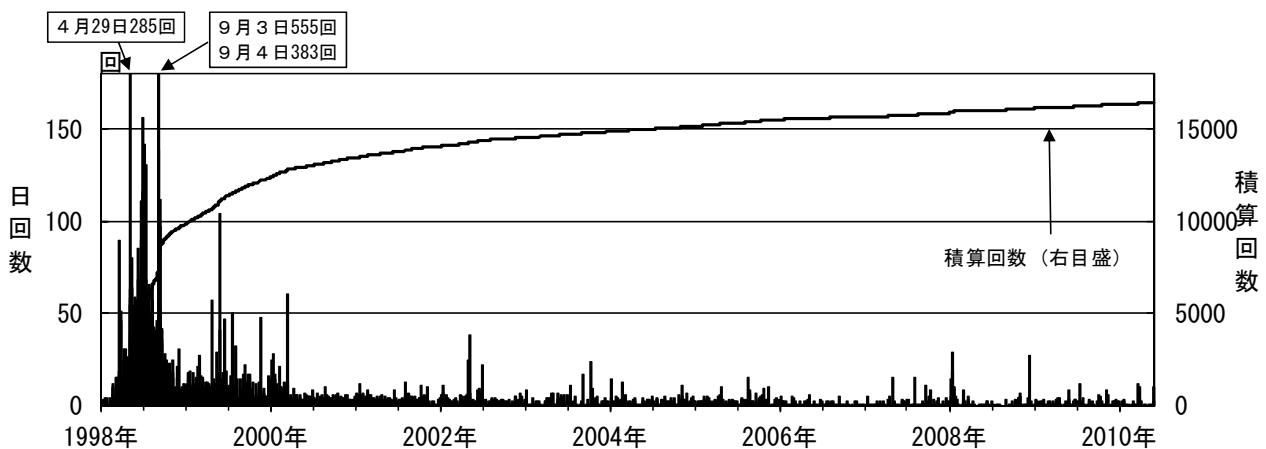
図 4※ 岩手山 日別地震回数（1998 年 1 月～2010 年 5 月）
