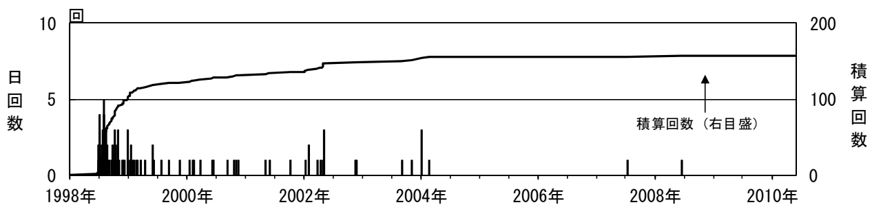
図 5※ 岩手山 日別微動回数（1998 年 1 月～2010 年 5 月）
