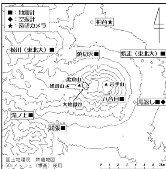
図 1 岩手山 観測点配置図
