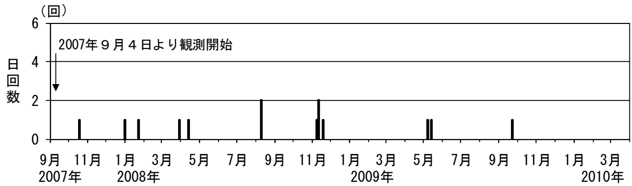
図 2※ 岩木山 日別地震回数（2007 年 9 月～2010 年 3 月）
