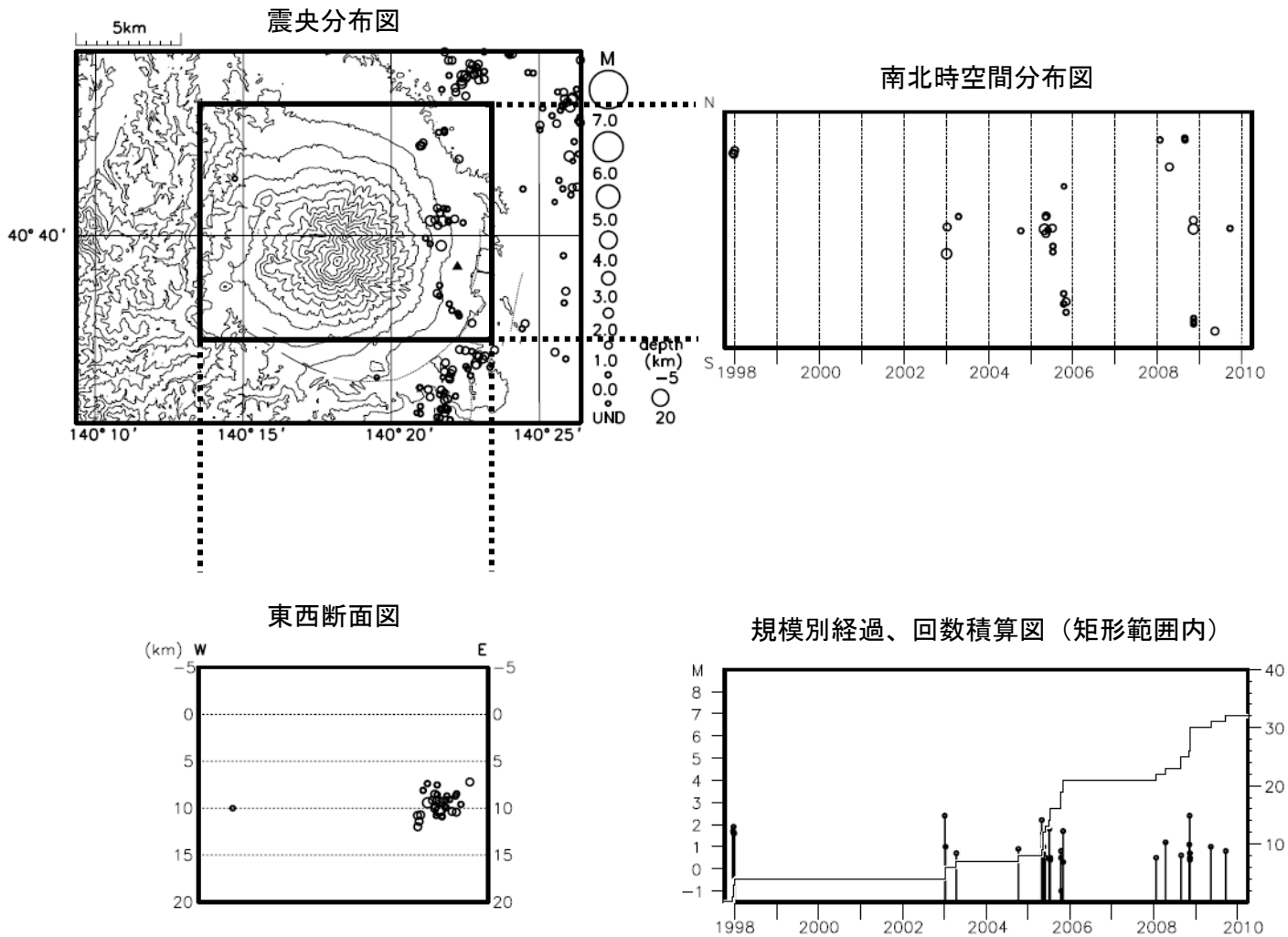
図 3※ 岩木山周辺の地震活動（1997 年 10 月～2010 年 3 月）
