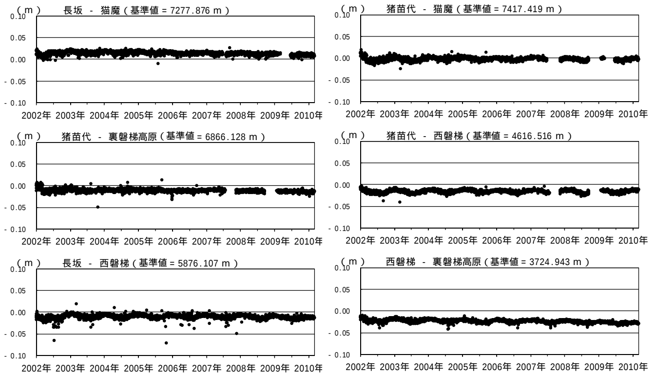
図6 磐梯山 GPS 基線長変化図（2002 年 1 月～2010 年 2 月）
