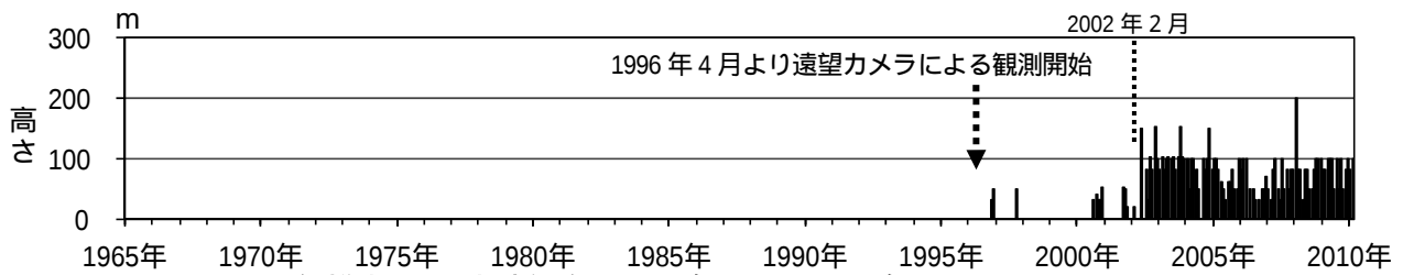
図 2 磐梯山 月最大噴気高（1996 年 4 月～2010 年 2 月）
