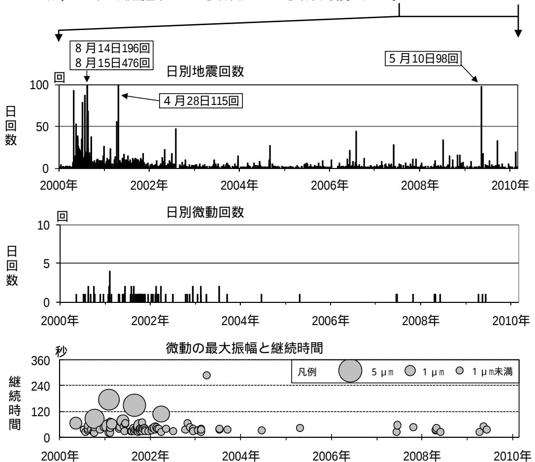
図 4 磐梯山 最近の地震と微動の活動経過図（2000 年 1 月～2010 年 2 月）
