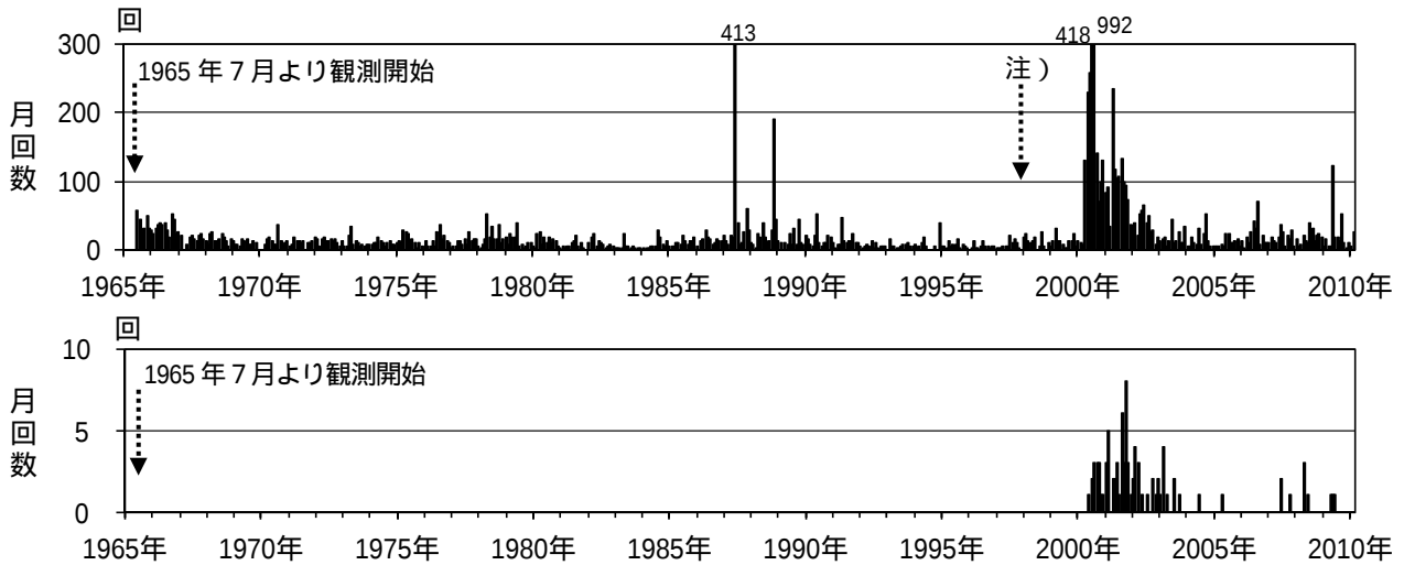
図 3 磐梯山 上段：月別地震回数(1965 年 7 月～2010 年 2 月)
