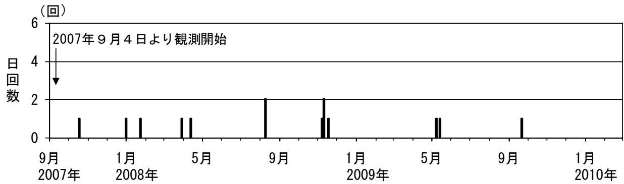
図 2※ 岩木山 日別地震回数（2007 年 9 月～2010 年 2 月）
