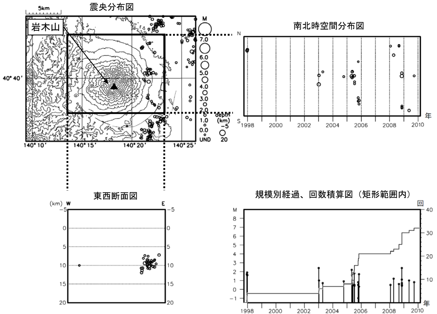
図 3※ 岩木山周辺の地震活動（1997 年 10 月～2010 年 2 月）
