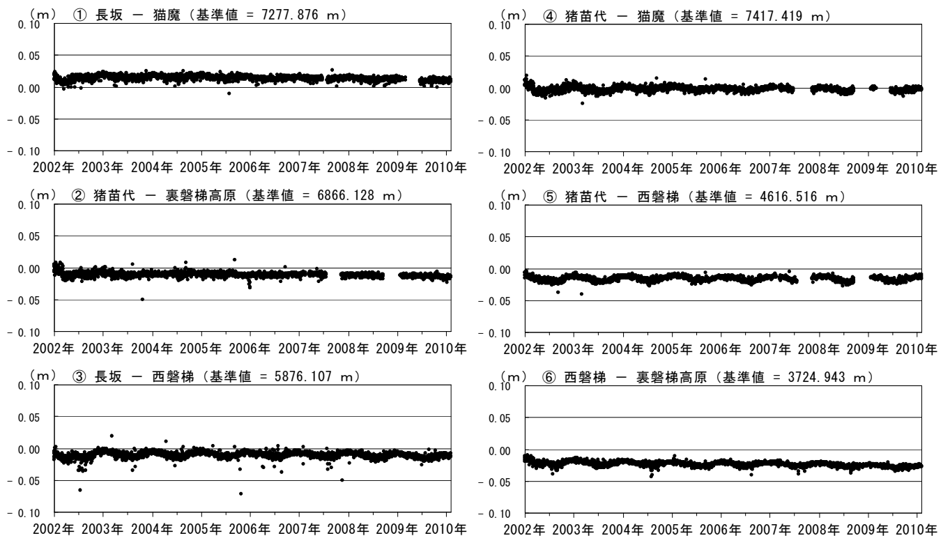
図6 磐梯山 GPS 基線長変化図（2002 年 1 月～2010 年 1 月）
