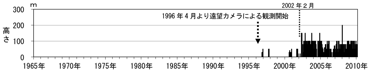
図 2 磐梯山 月最大噴気高（1996 年 4 月～2010 年 1 月）
