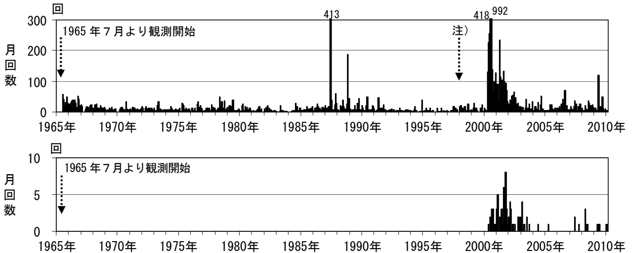
図 3 磐梯山 上段：月別地震回数（1965 年 7 月～2010 年 1 月）
