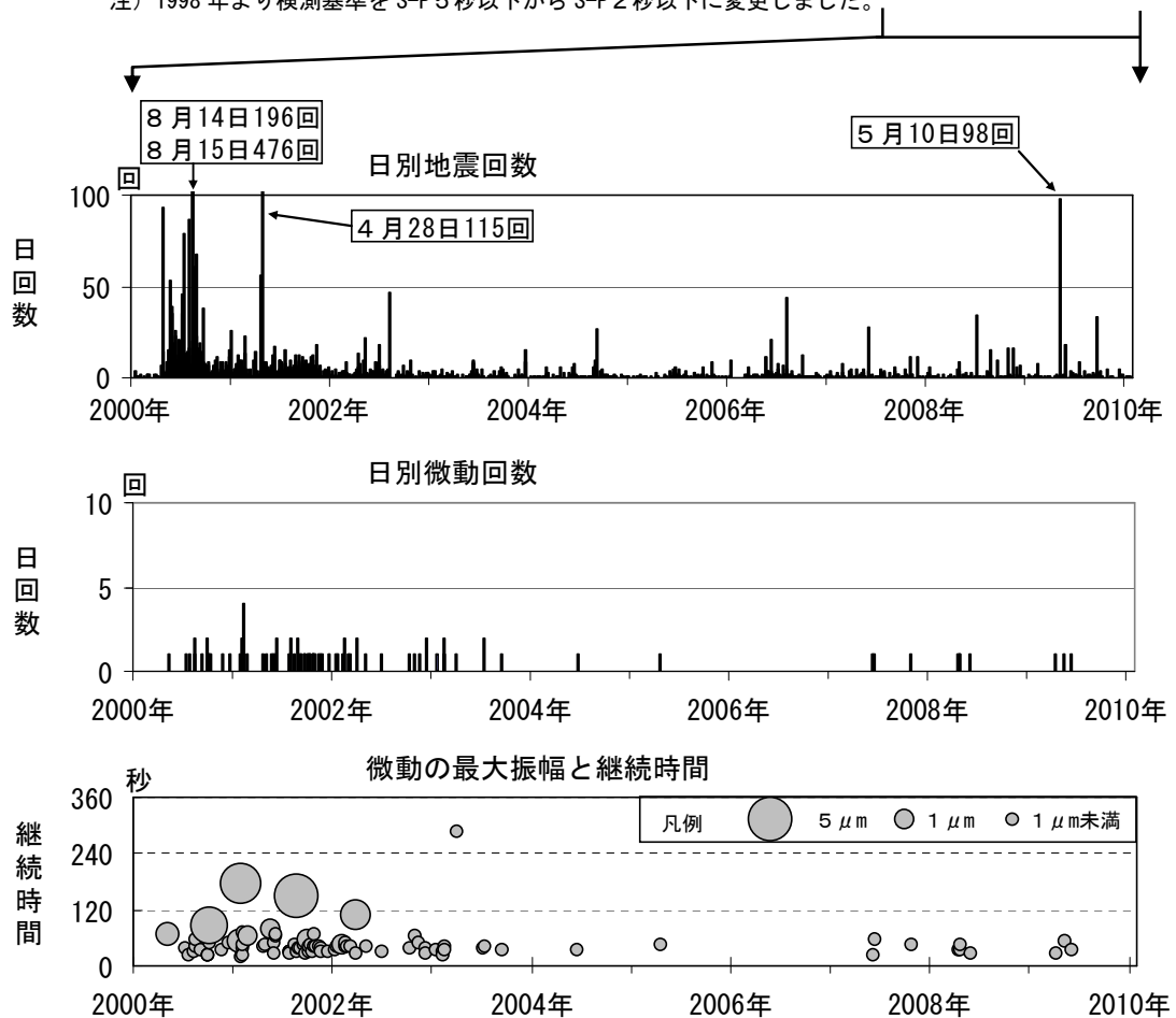
図 4 磐梯山 最近の地震と微動の活動経過図（2000 年 1 月～2010 年 1 月）
