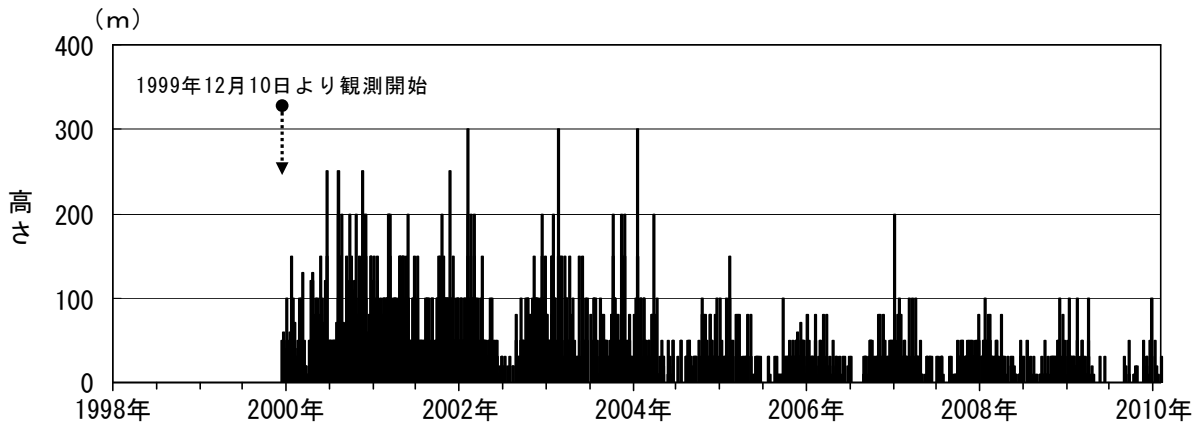
図 2 岩手山 日最大噴気の高さ（黒倉山）（1999 年 12 月～2010 年 1 月） 柏台遠望カメラで、1999 年 12 月 10 日より観測を開始しています。
