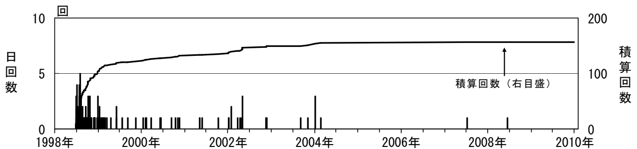
図 4※ 岩手山 日別微動回数（1998 年 1 月～2010 年 1 月）
