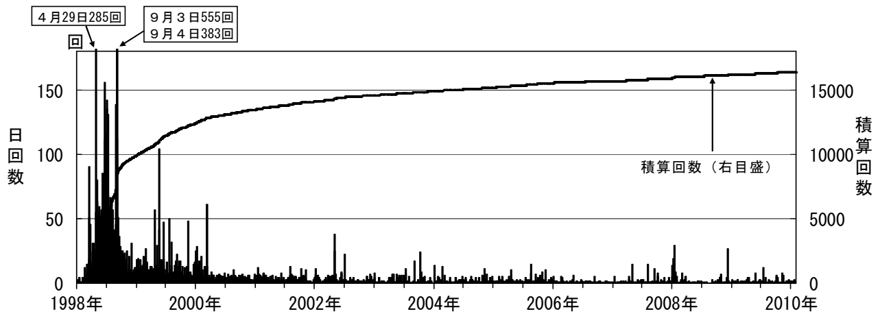
図 3※ 岩手山 日別地震回数（1998 年 1 月～2010 年 1 月）
