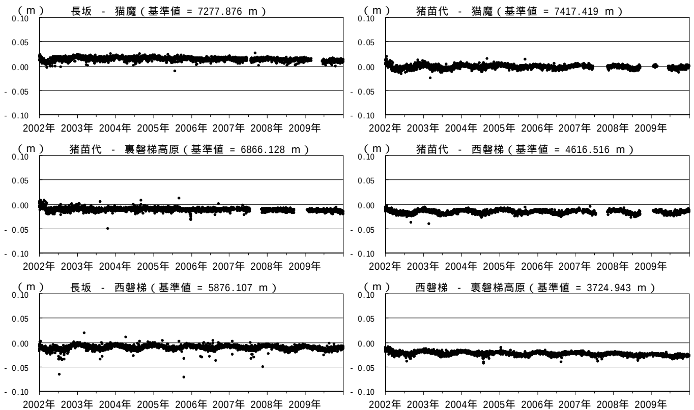
図6 磐梯山 GPS 基線長変化図（2002 年 1 月～2009 年 12 月）
