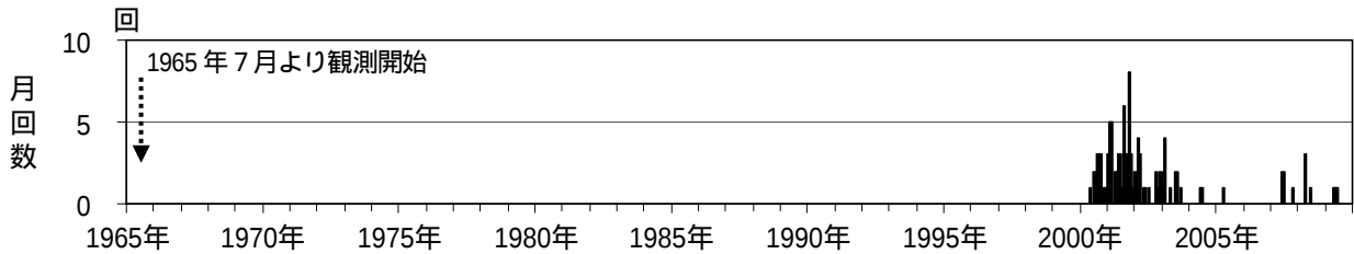
図3 磐梯山 上段：月別地震回数(1965年7月～2009年12月)
