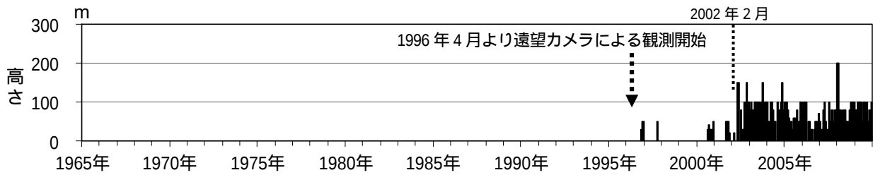
図2 磐梯山 月最大噴気高（1996年4月～2009年12月）
