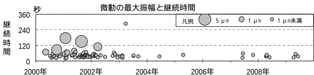
図4 磐梯山 最近の地震と微動の活動経過図（2000年1月～2009年12月）
