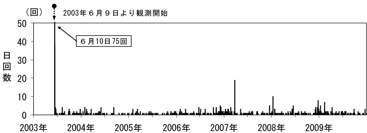
図5* 秋田駒ヶ岳 日別地震回数（2003年6月～2009年12月）
