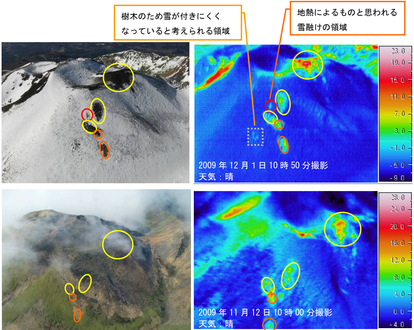
図4 秋田駒ヶ岳 女岳北東斜面の可視画像（左）と地表面温度分布 1) （右）（詳細）
