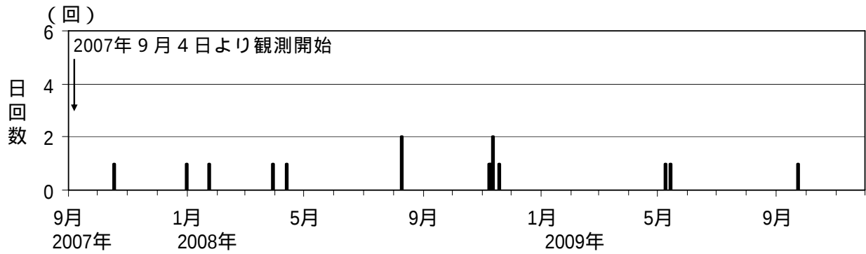
図2 岩木山 日別地震回数（2007年9月～2009年11月）
