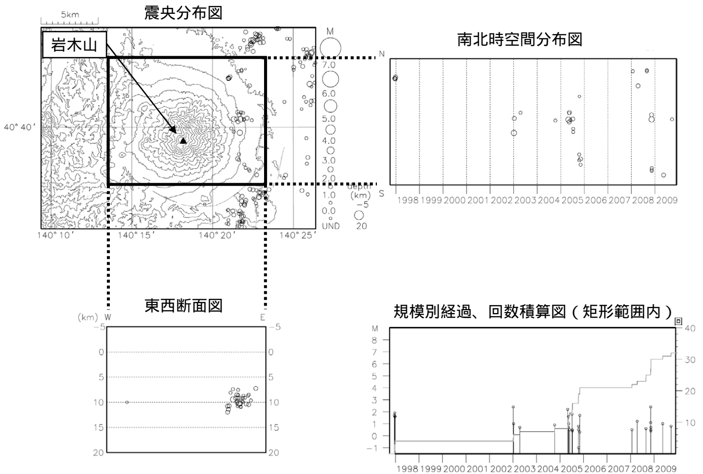
図3 岩木山周辺の地震活動（1997年10月～2009年11月）
