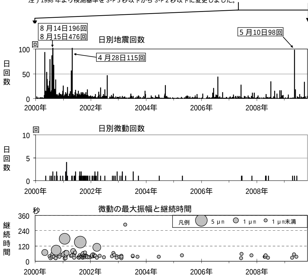
図4 磐梯山 最近の地震と微動の活動経過図（2000年1月～2009年10月）
