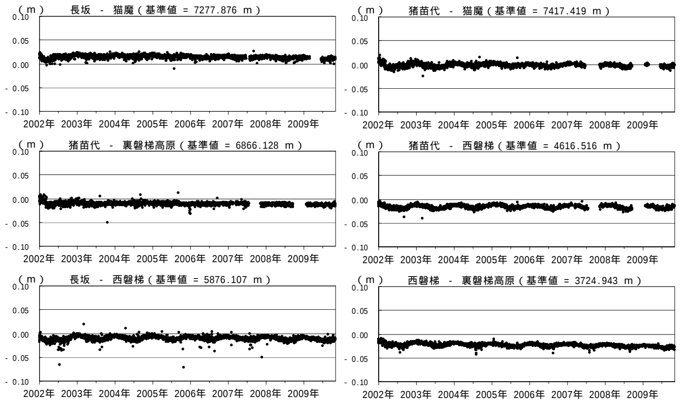
図6 磐梯山 GPS 基線長変化図（2002 年 1 月～2009 年 10 月）
