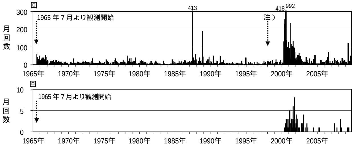
図3 磐梯山 上段：月別地震回数(1965年7月～2009年10月)
