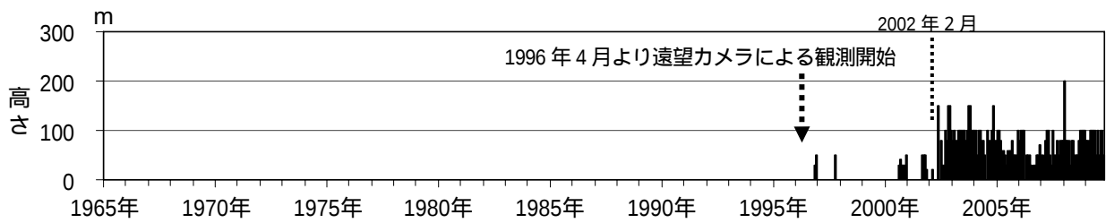
図2 磐梯山 月最大噴気高（1996年4月～2009年10月）
