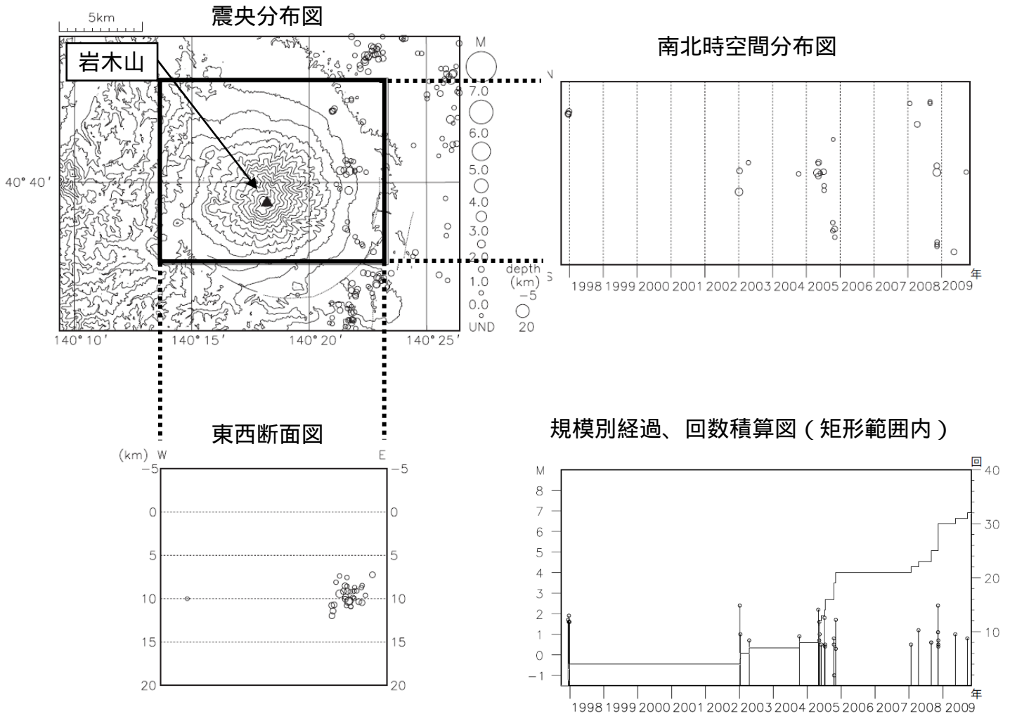
図3 岩木山周辺の地震活動（1997年10月～2009年10月）
