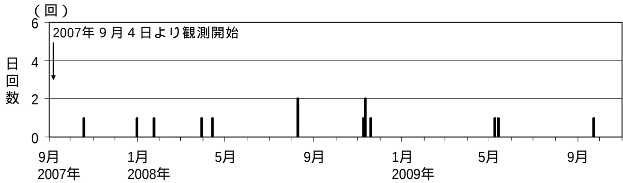
図2 岩木山 日別地震回数（2007年9月～2009年10月）
