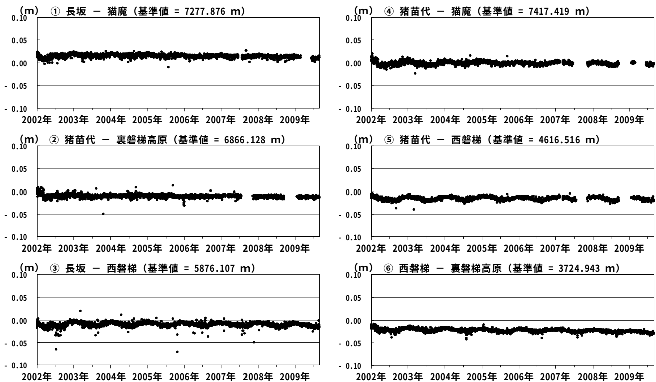
図6 磐梯山 GPS 基線長変化図 (2002 年 1 月～2009 年 8 月)
