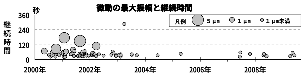
図4 磐梯山 最近の地震と微動の活動経過図(2000年1月～2009年8月)
