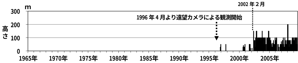
図2 磐梯山 月最大噴気高（1996年4月～2009年8月）
