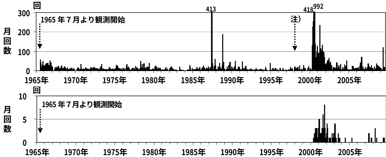
図3 磐梯山 上段：月別地震回数(1965年7月～2009年8月) 下段：月別微動回数(1965年7月～2009年8月)
