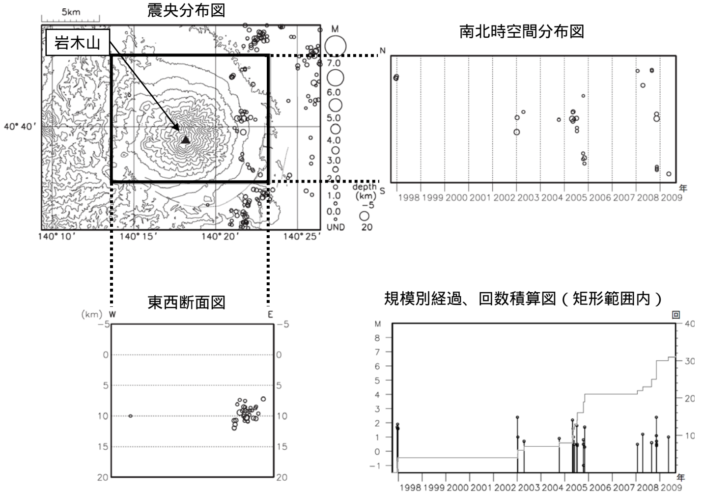
図 2 岩木山周辺の地震活動（1997 年 10 月～2009 年 8 月）
