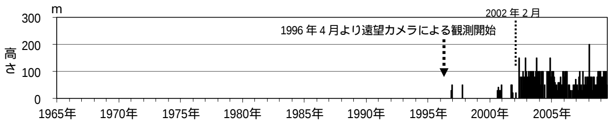
図2 磐梯山 月最大噴気高（1996年4月～2009年6月）
