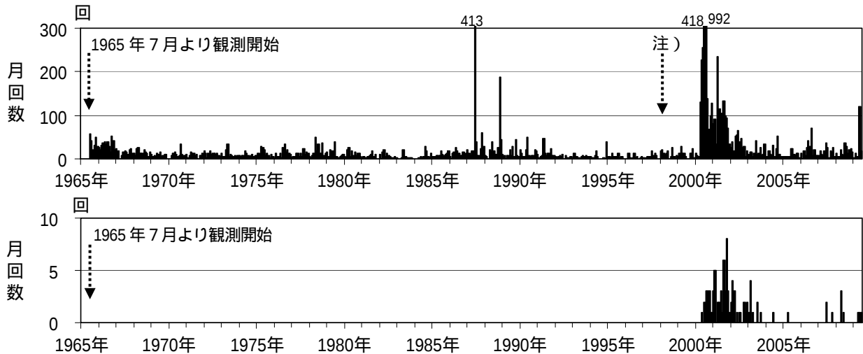
図3 磐梯山 上段：月別地震回数(1965年7月～2009年6月)
