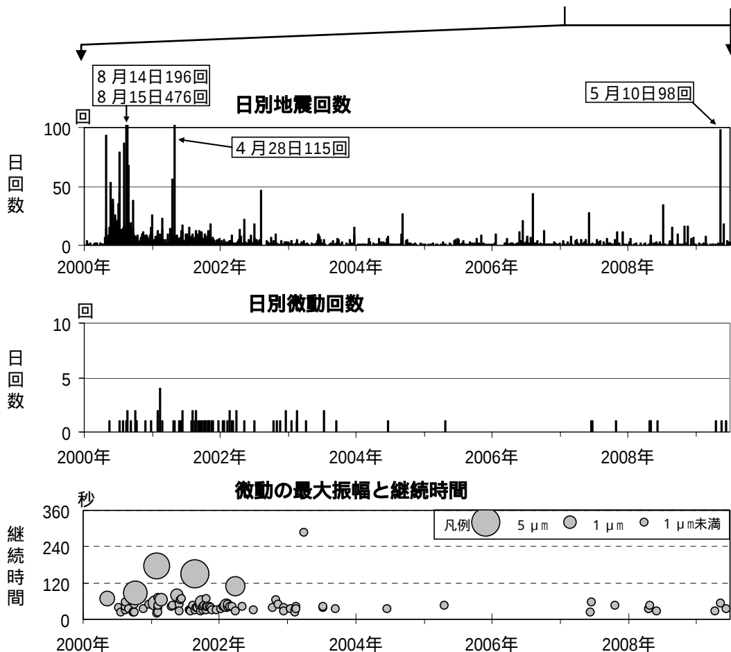
図4 磐梯山 最近の地震と微動の活動経過図(2000年1月～2009年6月)
