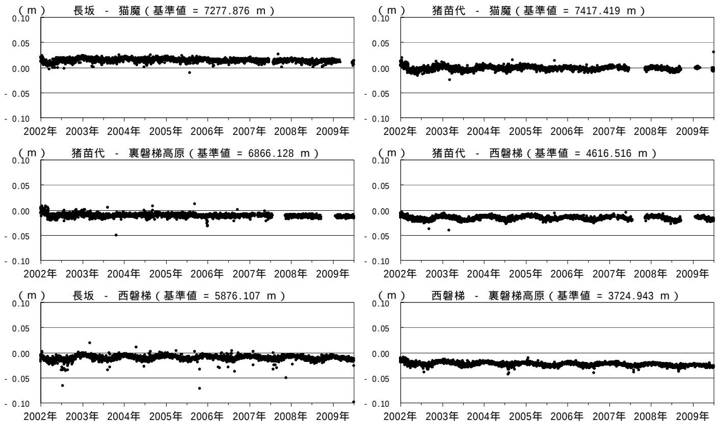
図 6 磐梯山 GPS 基線長変化図（2002 年 1 月～2009 年 6 月）
