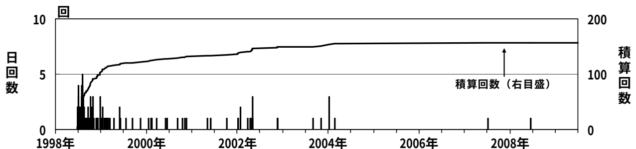
図4※ 岩手山 日別微動回数（1998 年 1 月～2009 年 6 月）
