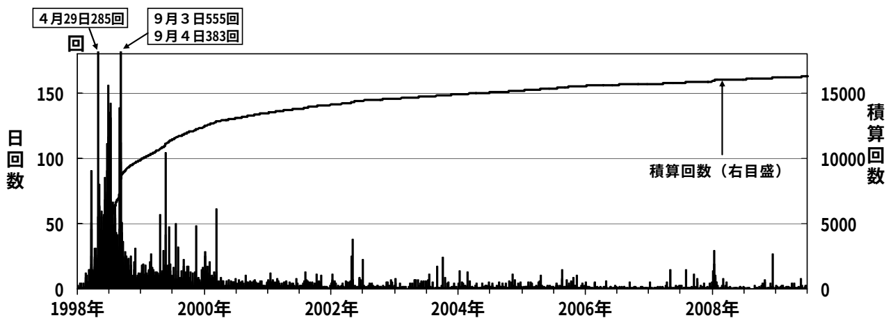
図3※ 岩手山 日別地震回数（1998 年 1 月～2009 年 6 月）
