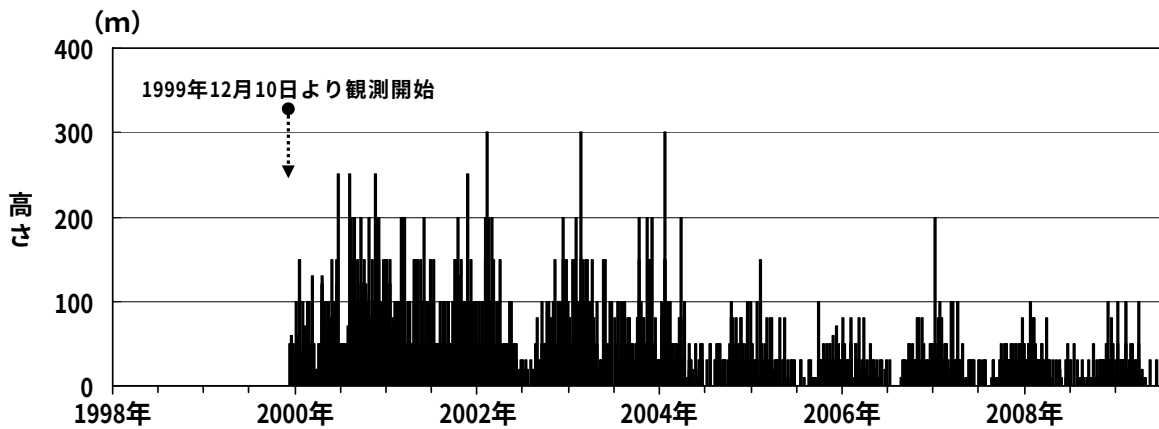
図2 岩手山 日最大噴気の高さ（黒倉山）（1999 年 12 月～2009 年 6 月）
