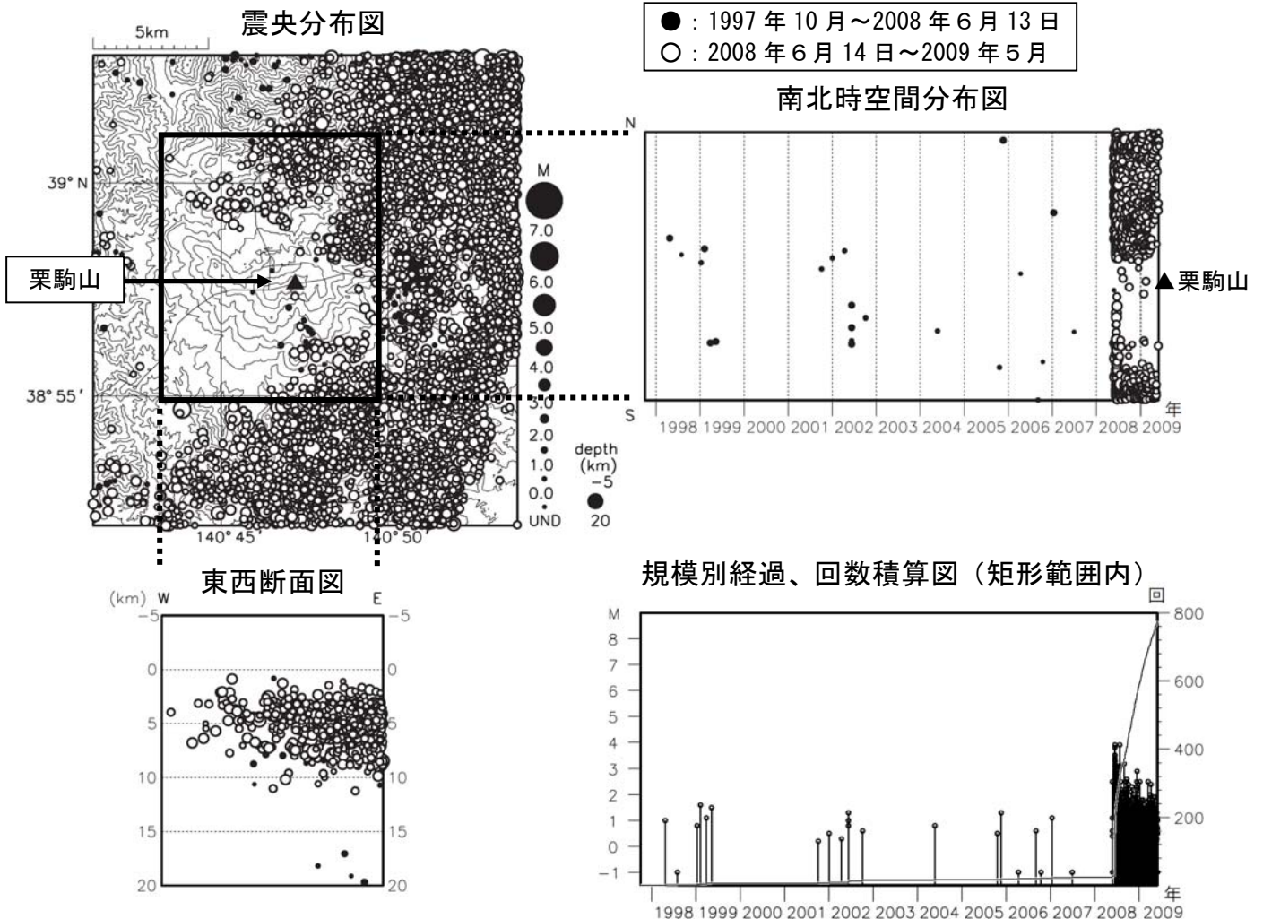
図 3※ 栗駒山周辺の地震活動（1997 年 10 月～2009 年 5 月）
