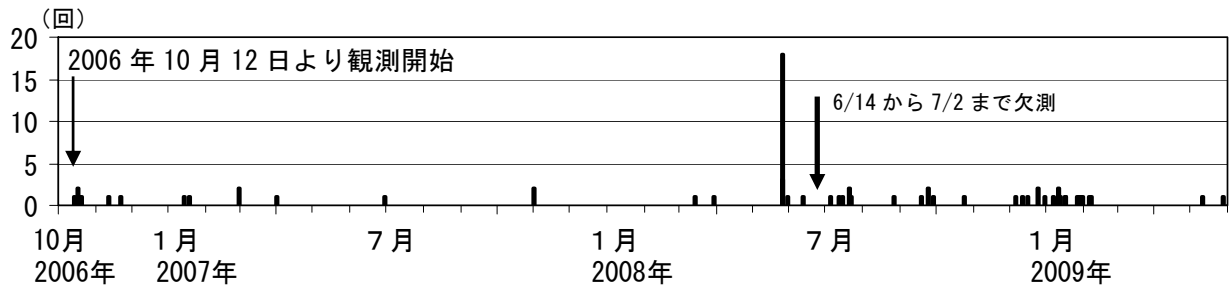
図 2 栗駒山 日別地震回数（2006 年 10 月～2009 年 5 月）
