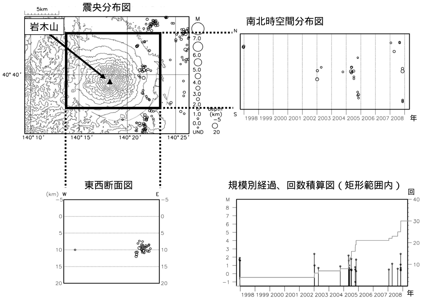
図 2 岩木山周辺の地震活動（1997 年 10 月～2009 年 4 月）
