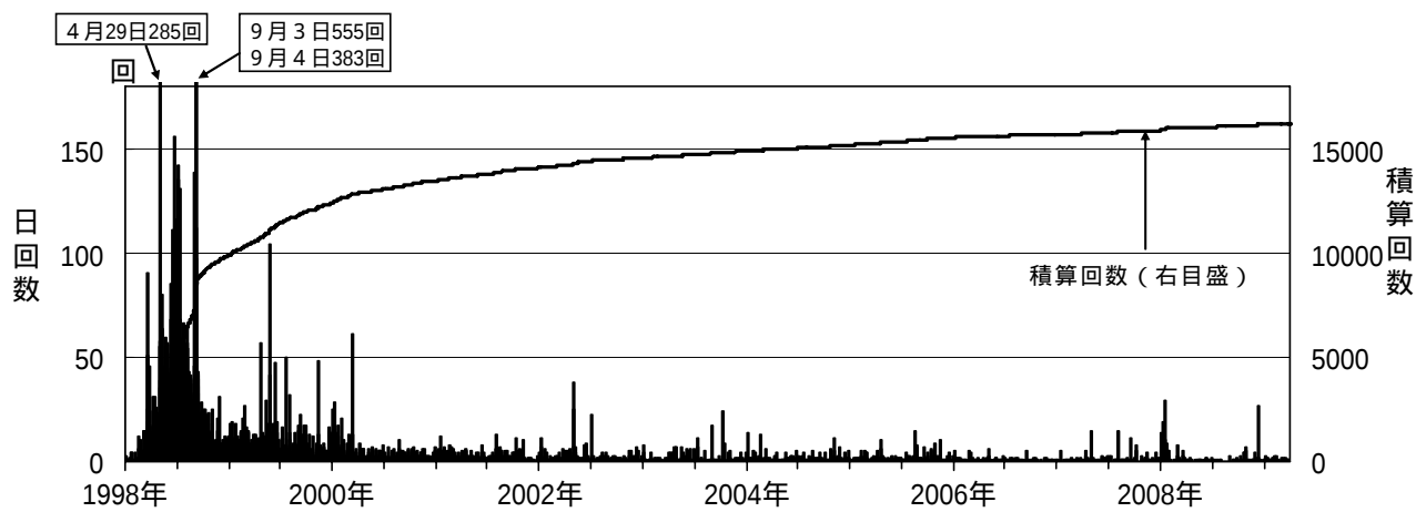
図3 岩手山 日別地震回数（1998 年 1 月～2009 年 3 月）
