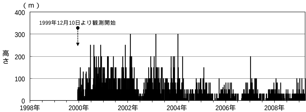
図2 岩手山 日最大噴気の高さ（黒倉山）（1999 年 12 月 10 日～2009 年 3 月）
