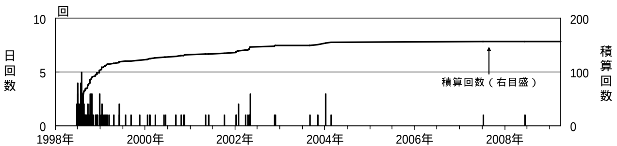
図4 岩手山 日別微動回数（1998 年 1 月～2009 年 3 月）
