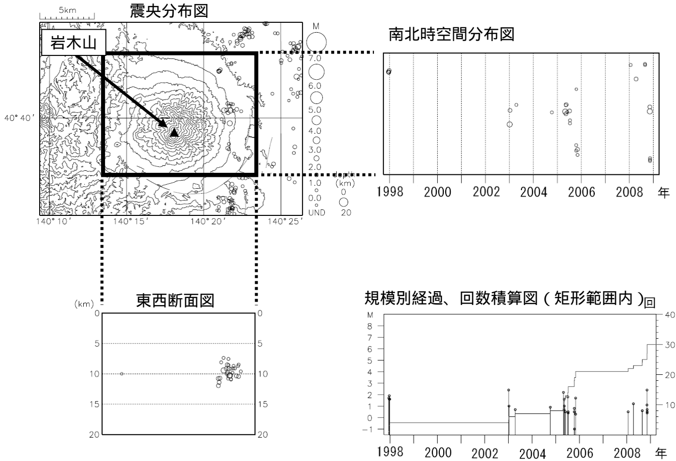
図 2 岩木山周辺の地震活動（1997 年 10 月～2009 年 3 月）
