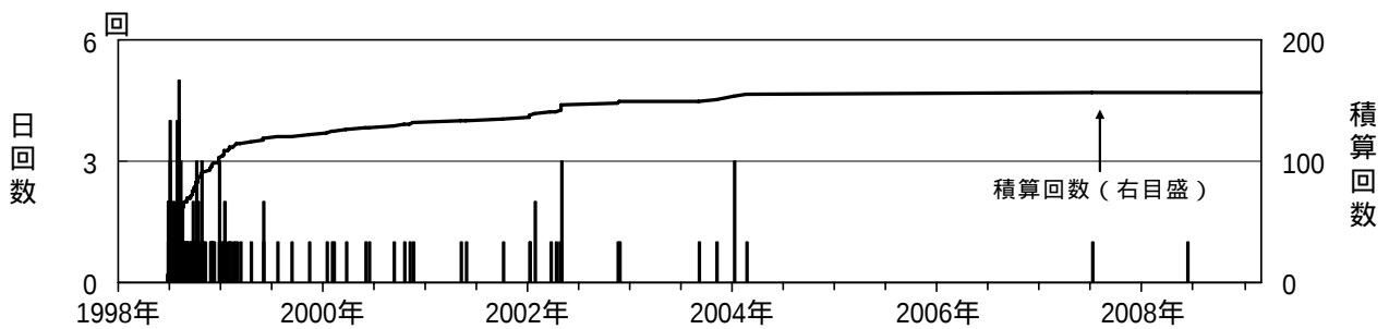
図3 岩手山 日別微動回数（1998年1月～2009年2月）
