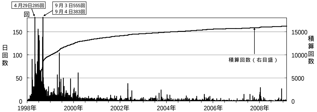
図2 岩手山 日別地震回数（1998年1月～2009年2月）
