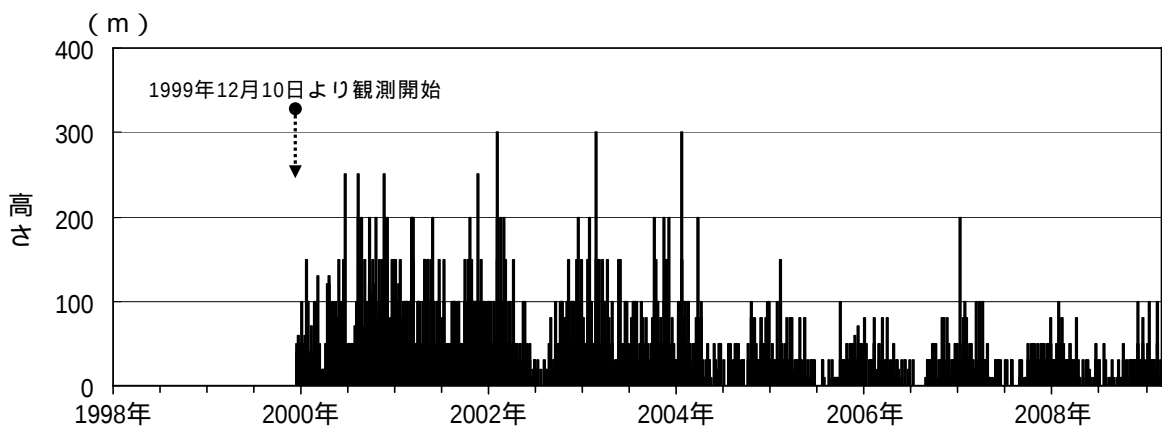
図4 岩手山 日最大噴気の高さ（黒倉山）（1999年12月10日～2009年2月）
