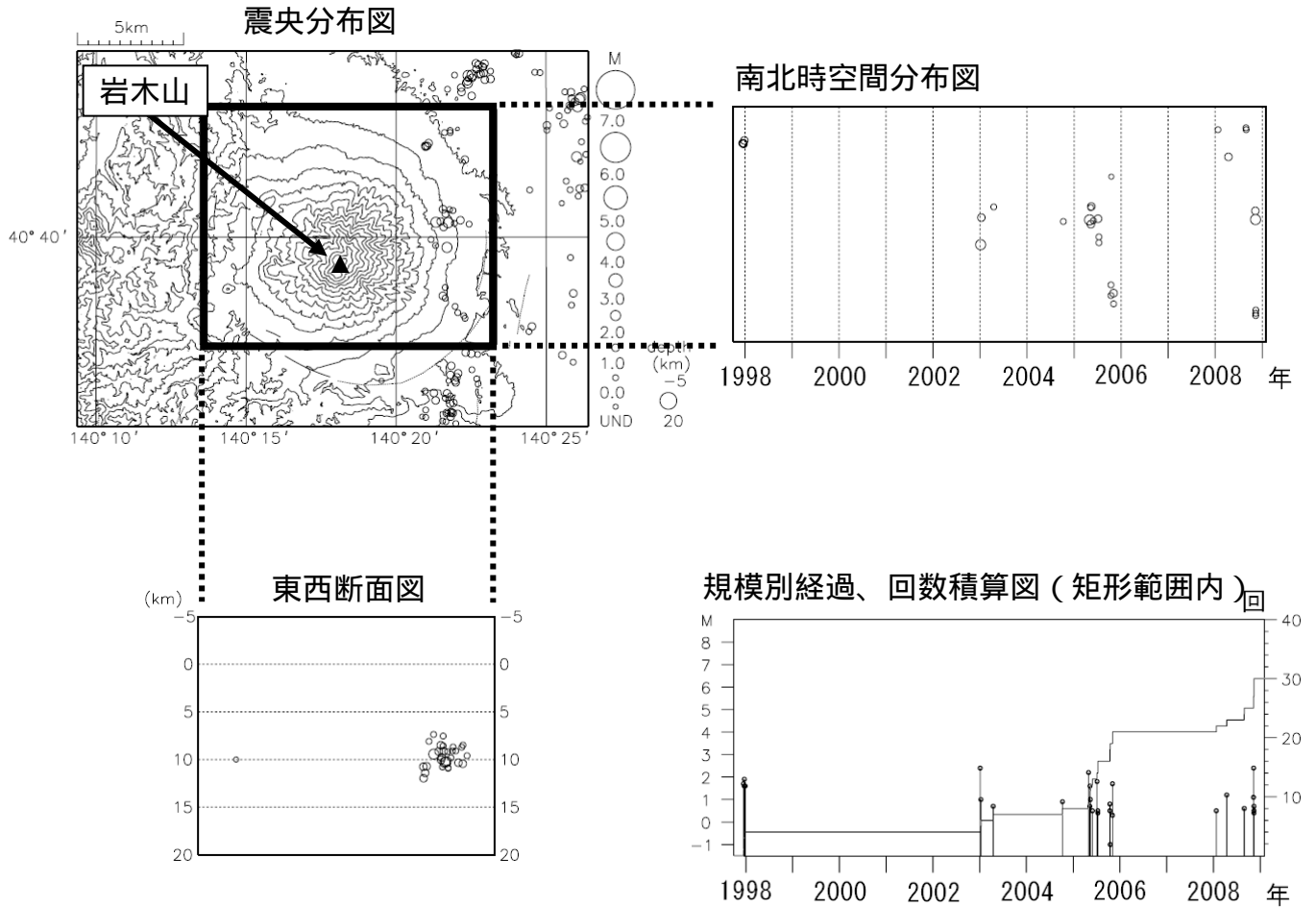
図 2 岩木山周辺の地震活動（1997 年 10 月～2009 年 1 月）
