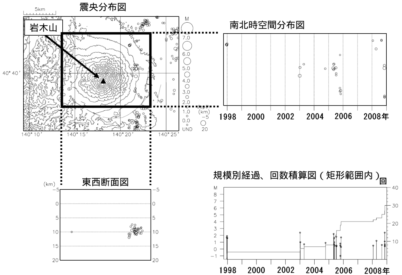
図 2 岩木山周辺の地震活動（1997 年 10 月～2008 年 12 月）
