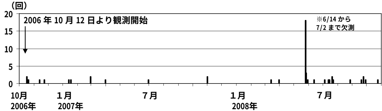
図 2 栗駒山 日別地震回数（2006 年 10 月～2008 年 10 月）
