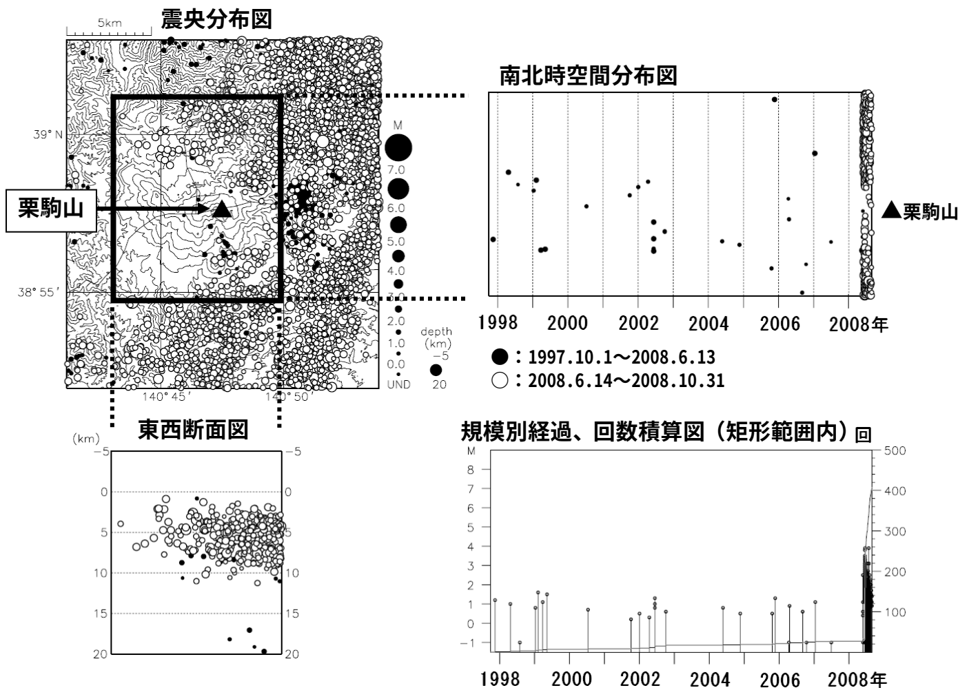
図 3※ 栗駒山周辺の地震活動（1997 年 10 月～2008 年 10 月）
