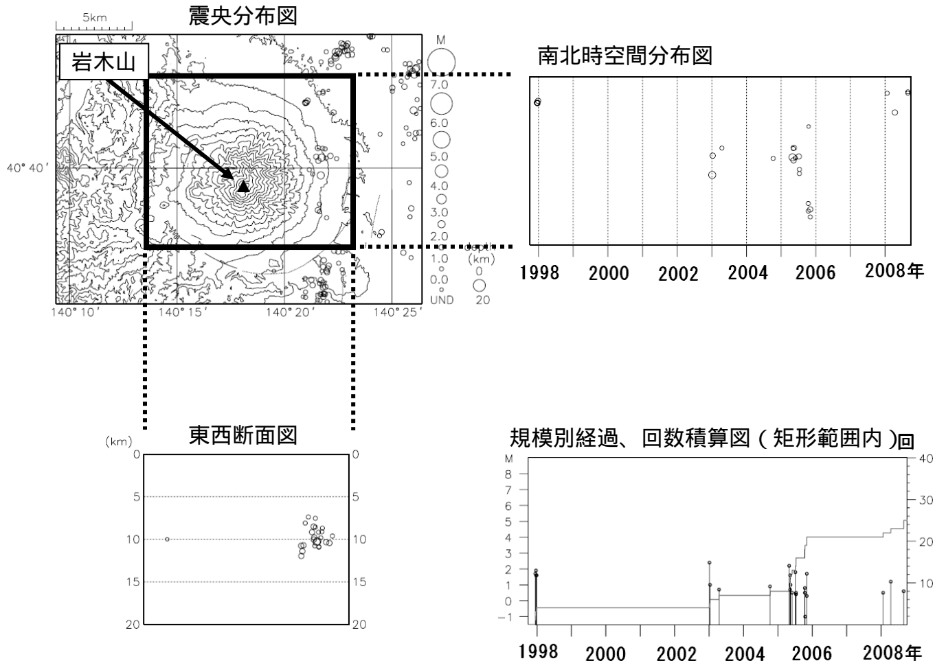
図 2 岩木山周辺の地震活動（1997 年 10 月～2008 年 9 月）
