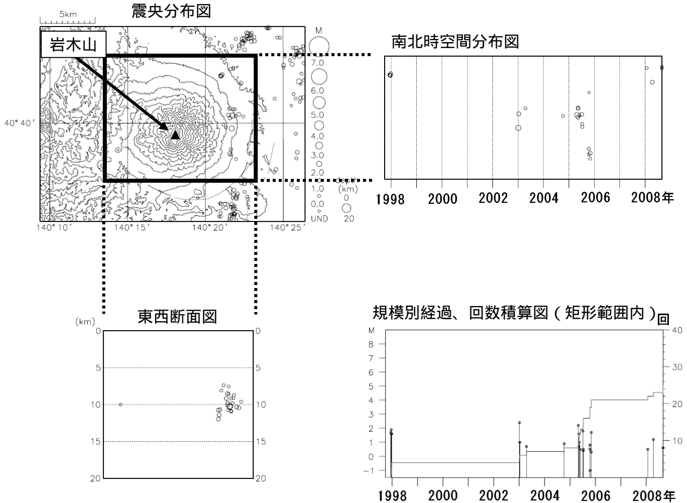
図 2 岩木山周辺の地震活動（1997 年 10 月～2008 年 8 月）
