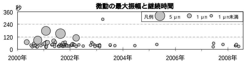
図 4 磐梯山 日別地震回数、日別微動回数、微動の振幅と継続時間 (2000 年 1 月～2008 年 7 月)
