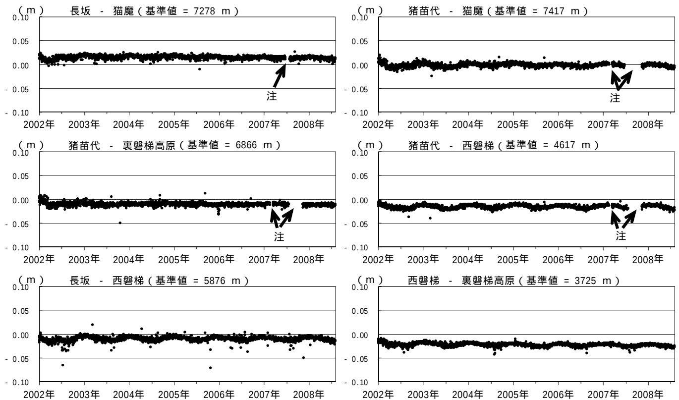
図 6 磐梯山 GPS 基線長変化図（2002 年 1 月～2008 年 7 月）
