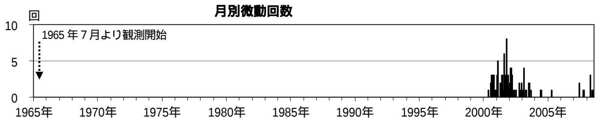
図 3 磐梯山 月別地震回数、月別微動回数(1965 年 7 月～2008 年 7 月)
