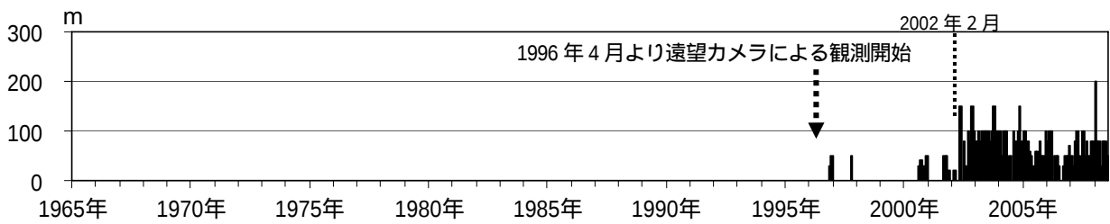
図 2 磐梯山 月最大噴気高（1996 年 4 月～2008 年 7 月）
