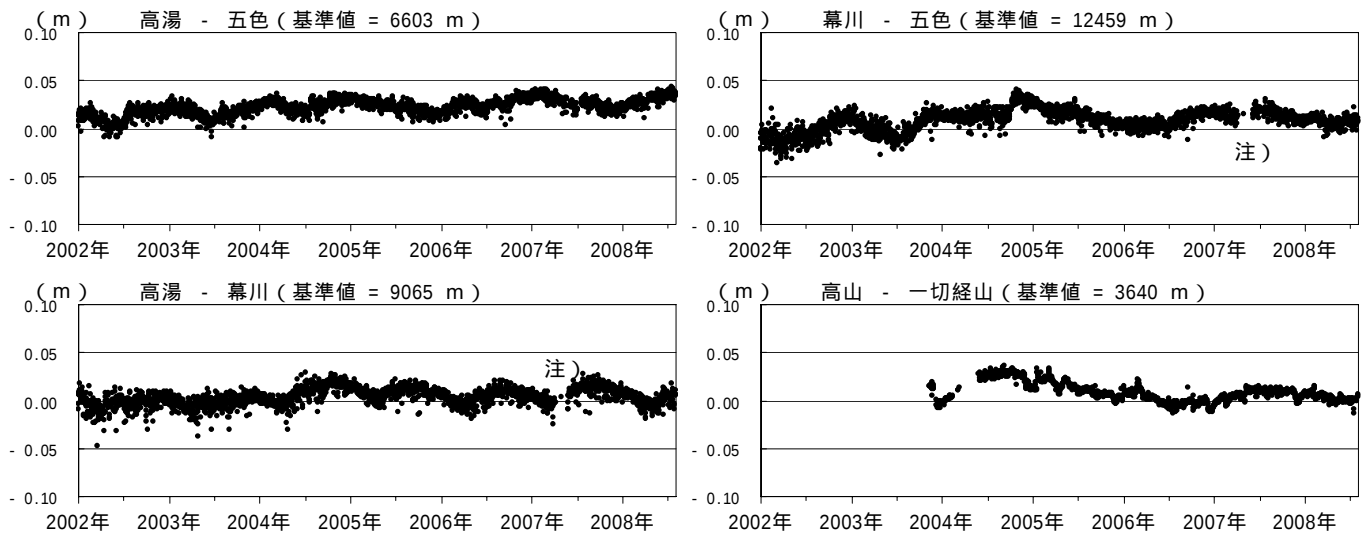
図 5 吾妻山 GPS 基線長変化図（2002 年 1 月～2008 年 7 月）
