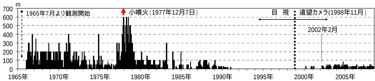
図2 吾妻山 月別最大噴気（噴煙）高（1965 年 7 月～2008 年 7 月）
